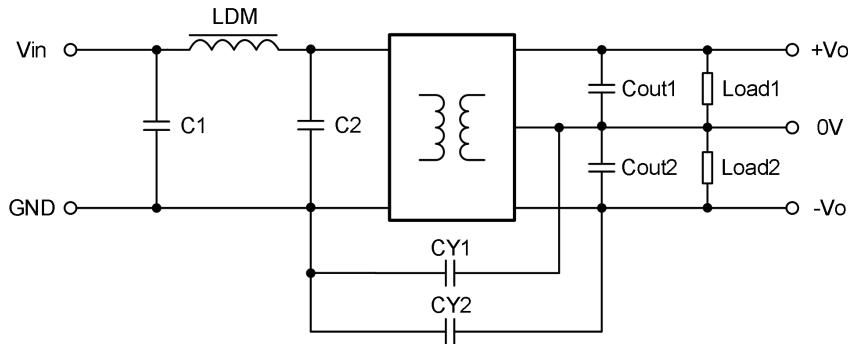
图 2 EMC 推荐电路图
