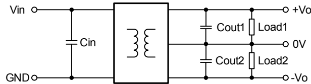
图 1 双路应用电路图
