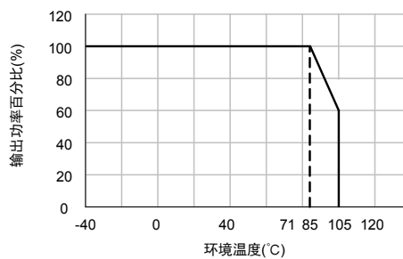
环境温度降额曲线图
