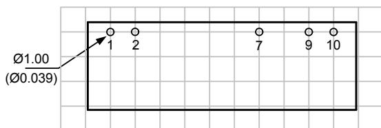
PCB丝印图(俯视图)
