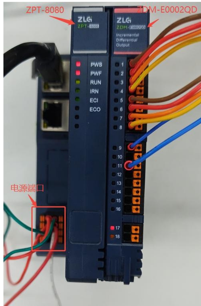
图 5.1 设备接线图
