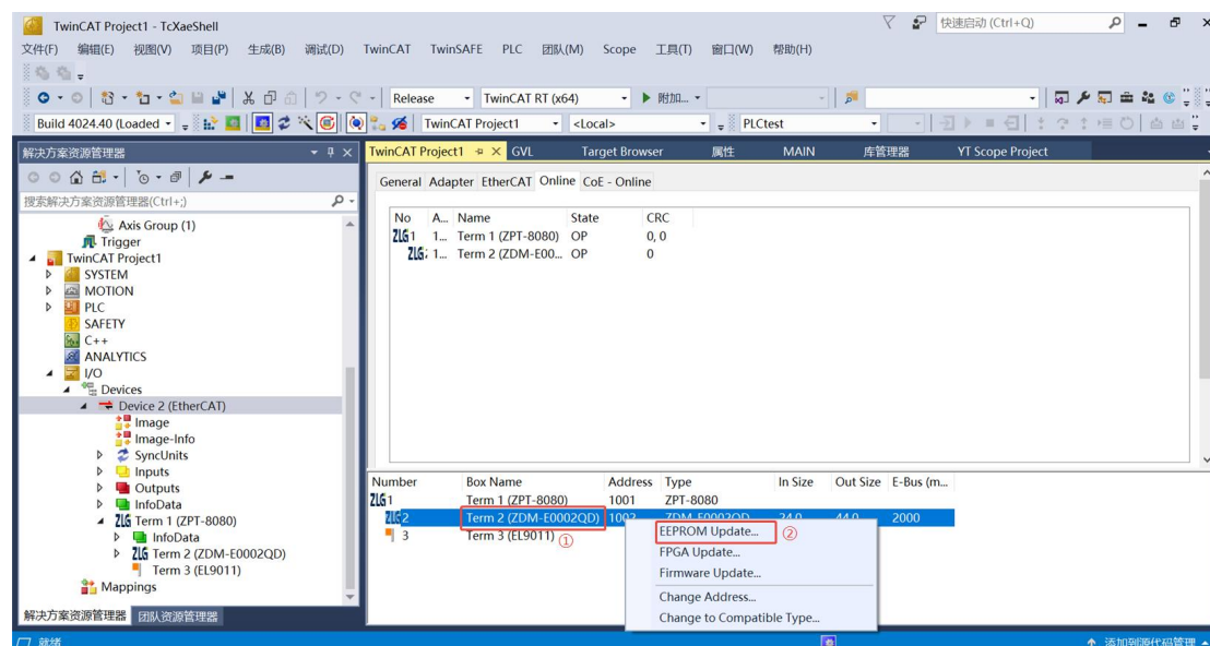
图 6.2 选择设备更新 EEPROM
