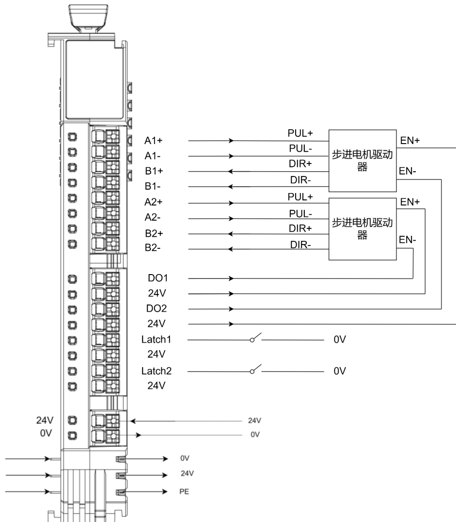
图 3.1 ZDM-E0002QD 模块接线图
