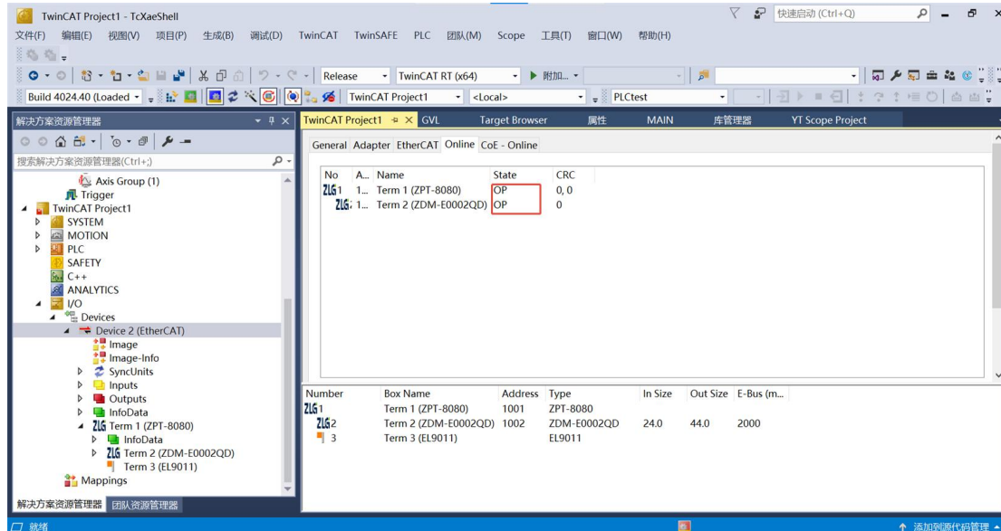
图 5.14 从站设备工作状态界面
