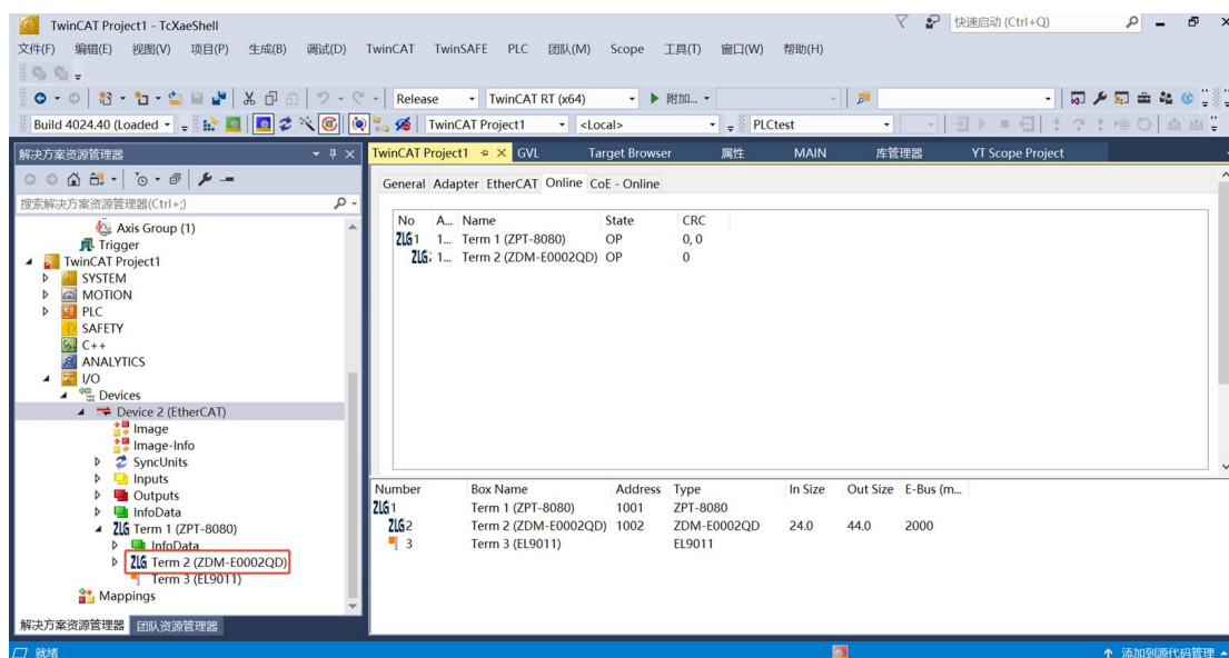
图 5.13 设备扫描成功界面
