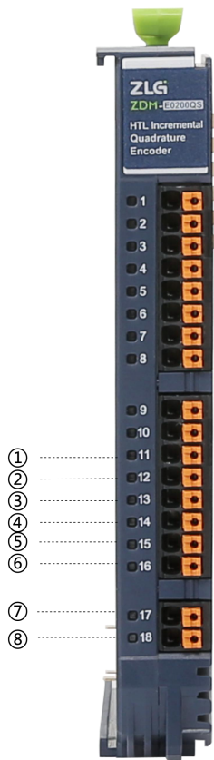
图 2.2 指示灯面板
