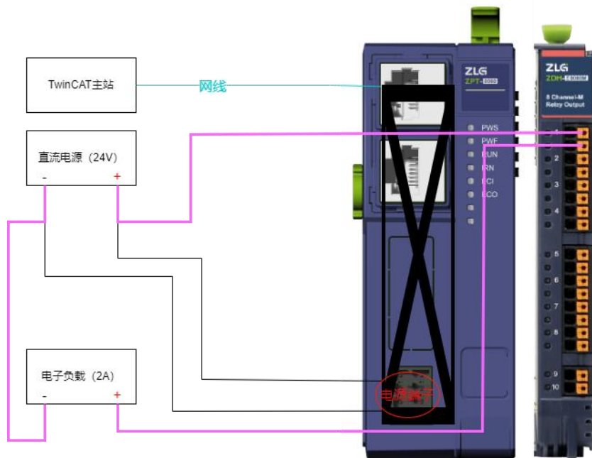
图 2 试验配置框图
