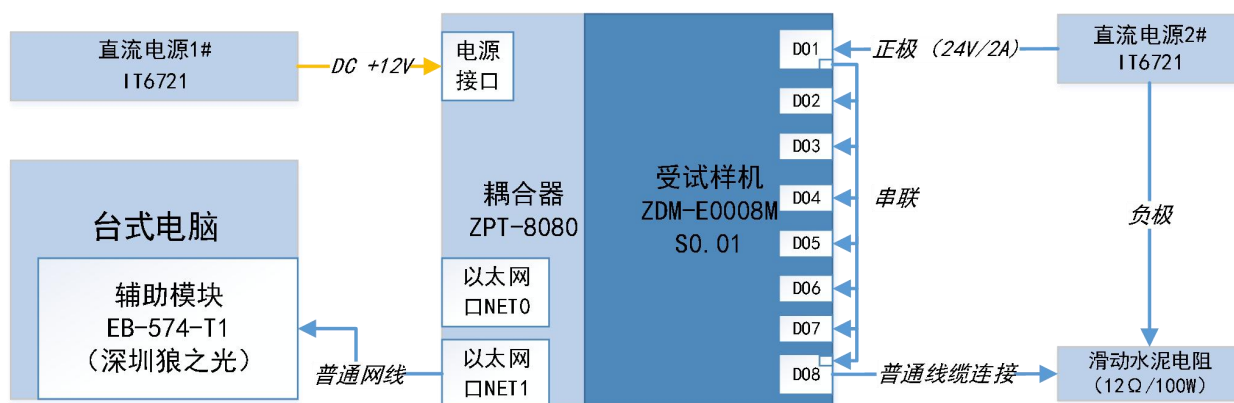
图 1 试验配置示意图
