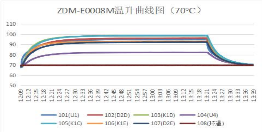
图 10 温升试验曲线（70℃）
