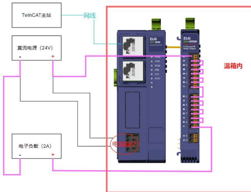
图 5 试验配置框图
