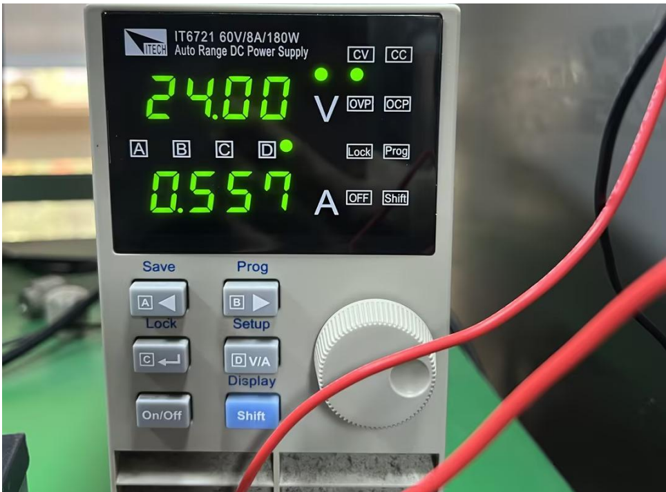
图 7 样机电压电流正常
