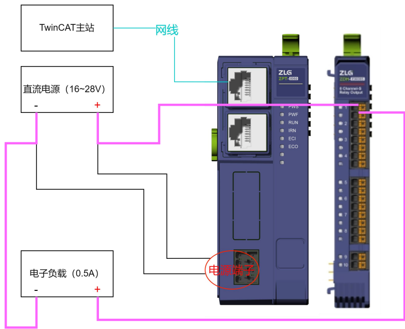
图 2 试验配置框图
