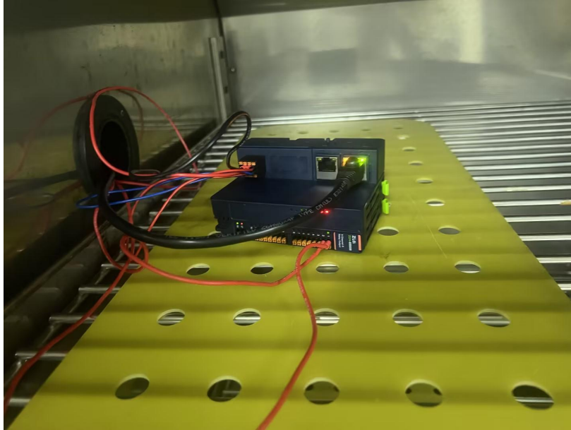
图 3 样机环境试验
