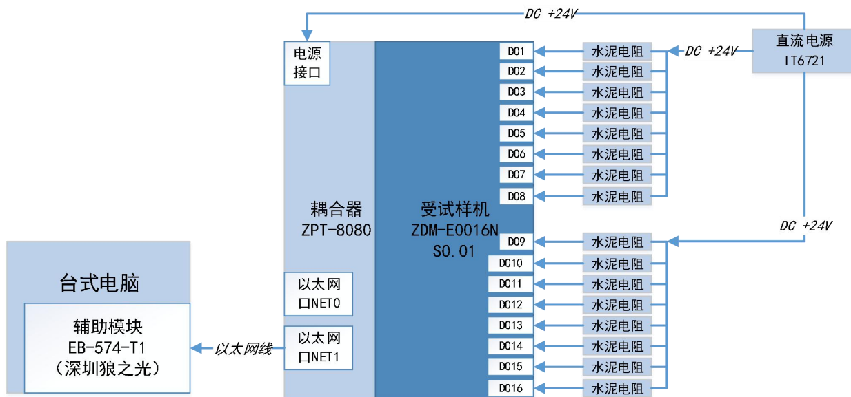
图 1 试验配置示意图
