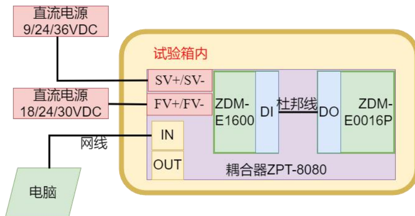
图 2 试验配置框图
