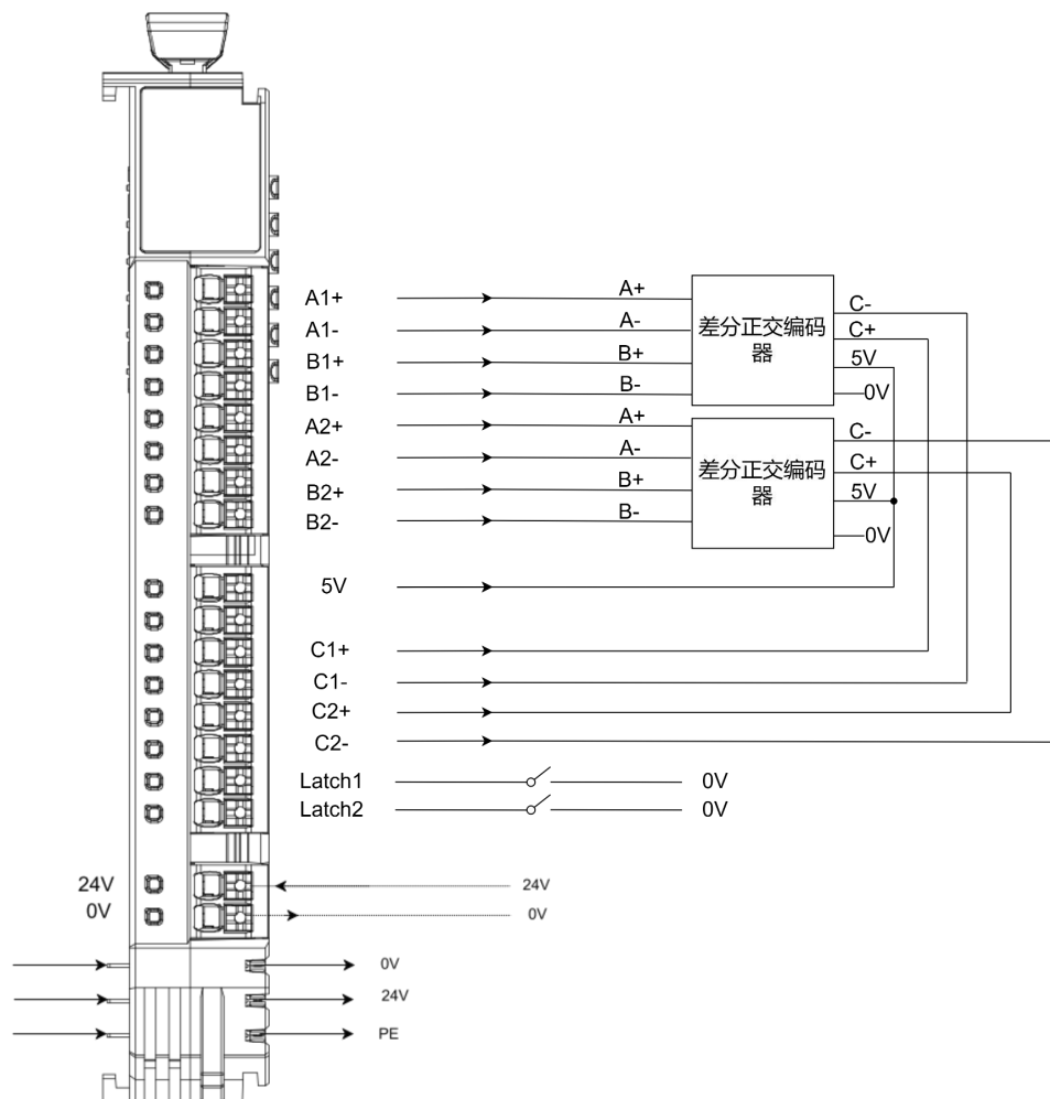
图 3.1 ZDM-E0200QD 模块接线图
