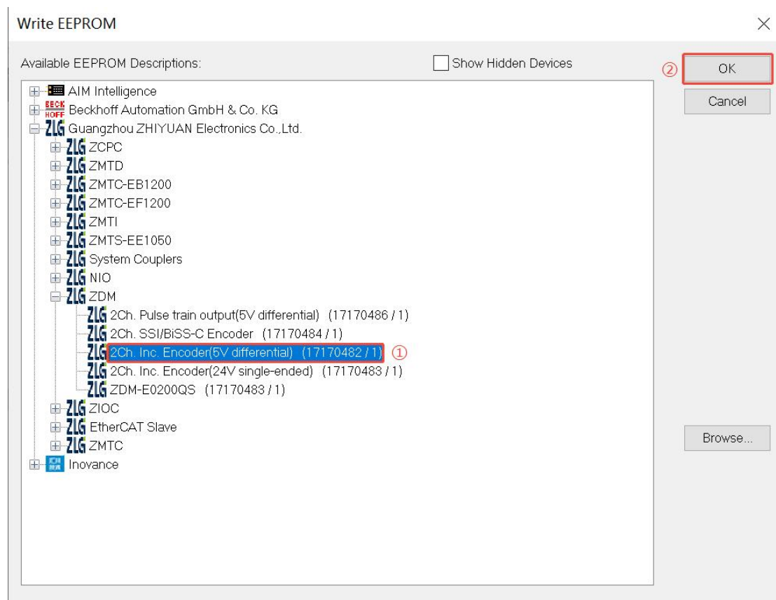
图 6.3 烧录 ESI 文件至 EEPROM
