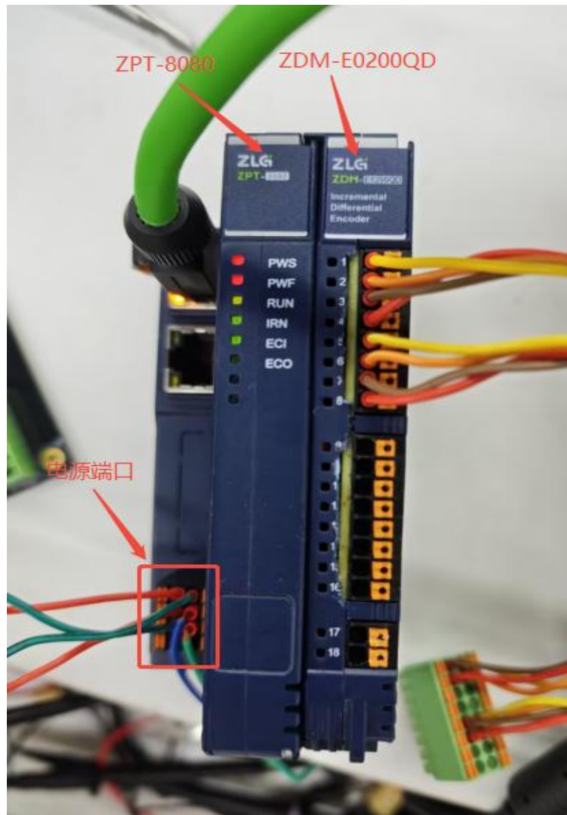
图 5.1 设备接线图
