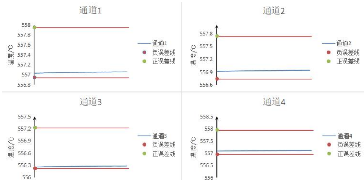
图 7 样机在低温试验时第二次启动运行检查功能正常 (24VDC 供电)
