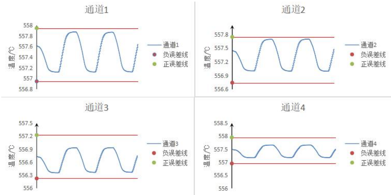
图 15 样机在温度变化试验时功能正常（24VDC 供电）
