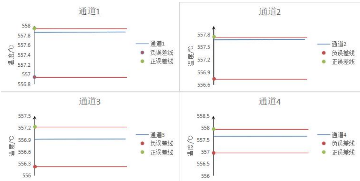
图 10 样机在高温试验时第二次启动运行检查功能正常（24VDC 供电）
