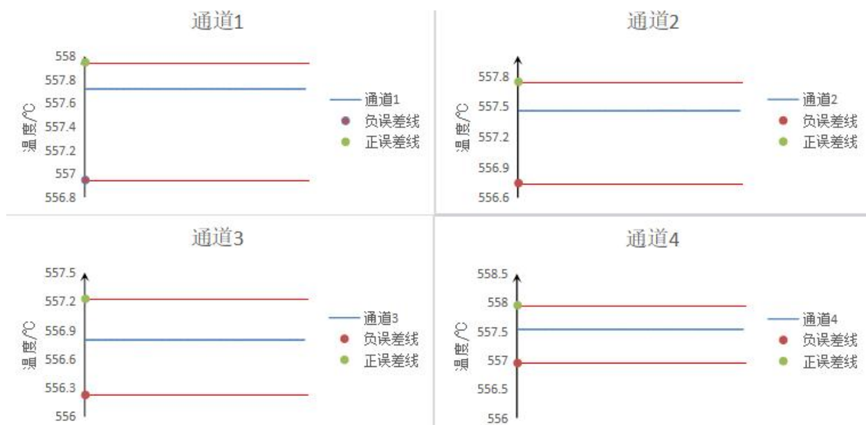
图 13 样机在湿热试验时第二次启动运行检查功能正常 (18VDC 供电)
