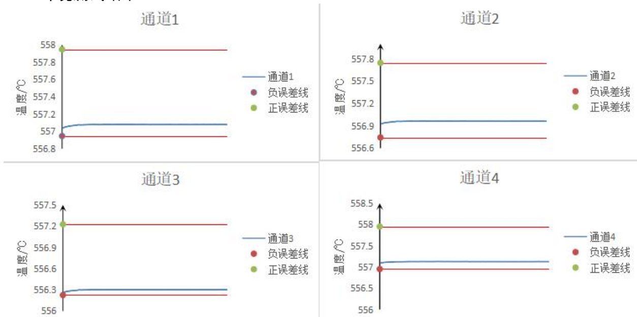
图 6 样机在低温试验时第一次启动运行检查功能正常 (18VDC 供电)
