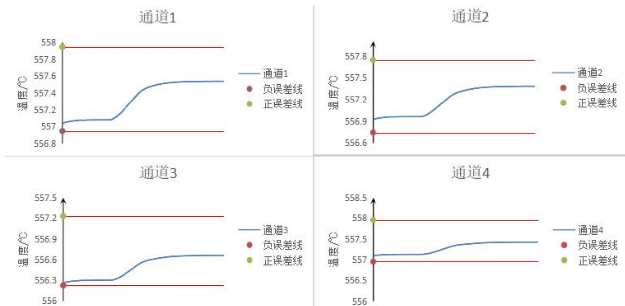
图 8 样机在低温试验时第三次启动运行检查功能正常 (30VDC 供电)
