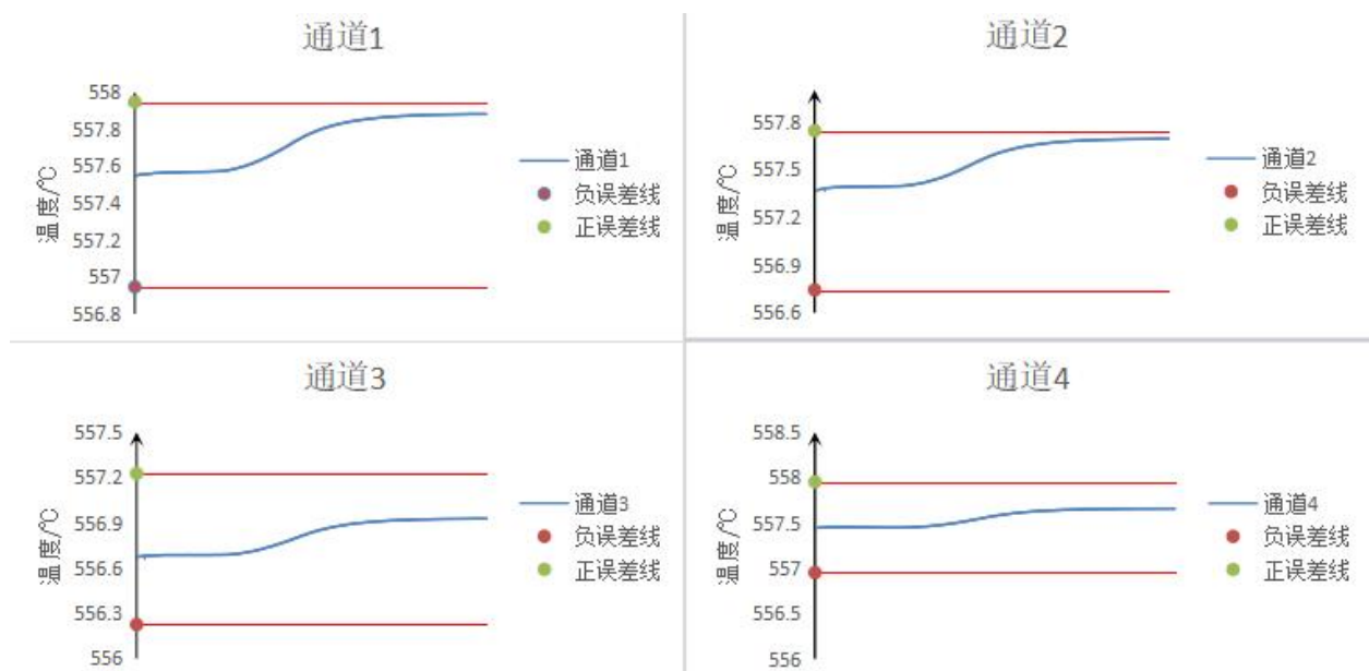
图 9 样机在高温试验时第一次启动运行检查功能正常 (30VDC 供电)
