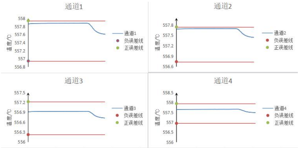
图 11 样机在高温试验时第三次启动运行检查功能正常（18VDC 供电）
