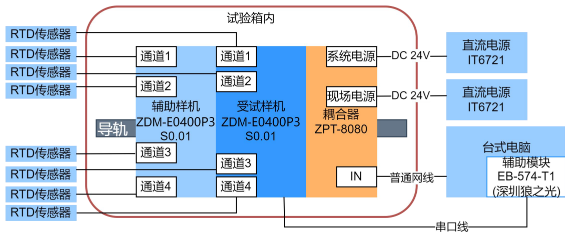
图 2 试验配置框图
