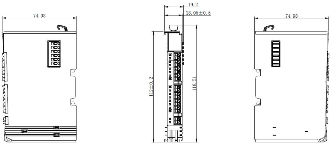
图 4.1 ZDM-E0800I 产品尺寸
