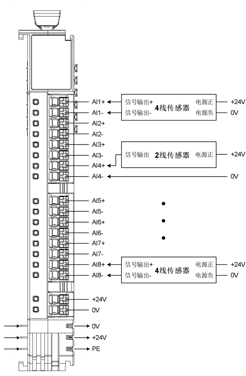
图 3.1 ZDM-E0800I 模块接线图
