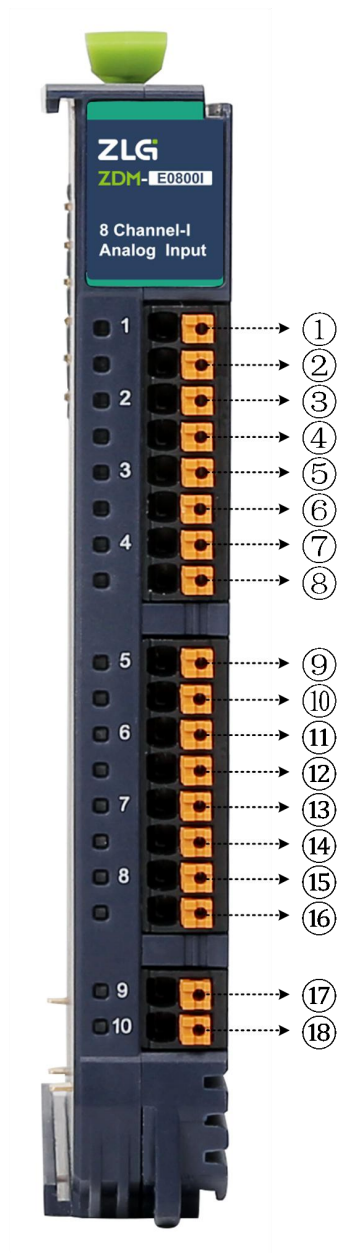
图 2.3 接线端子序号
