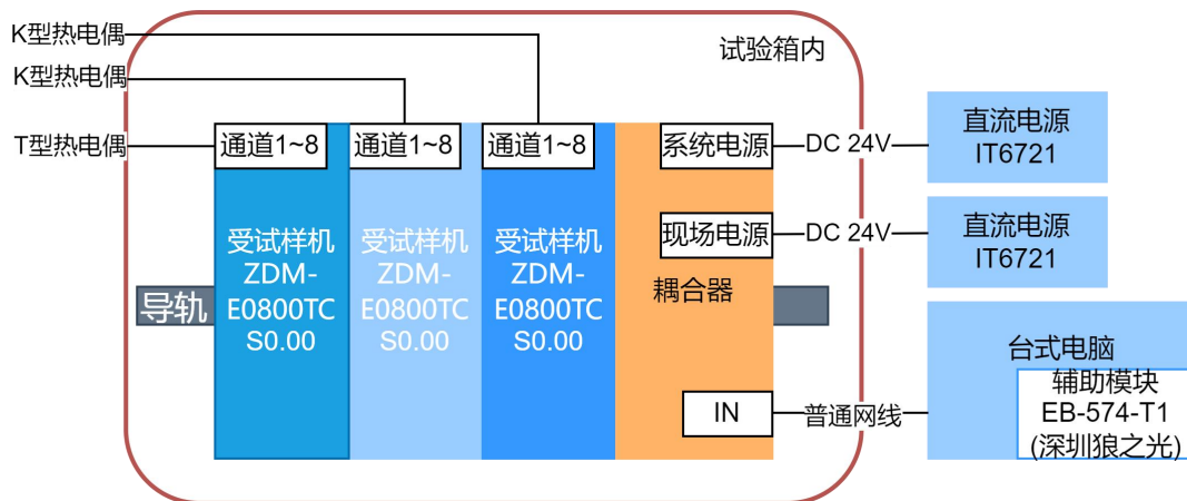
图 2 试验配置框图
