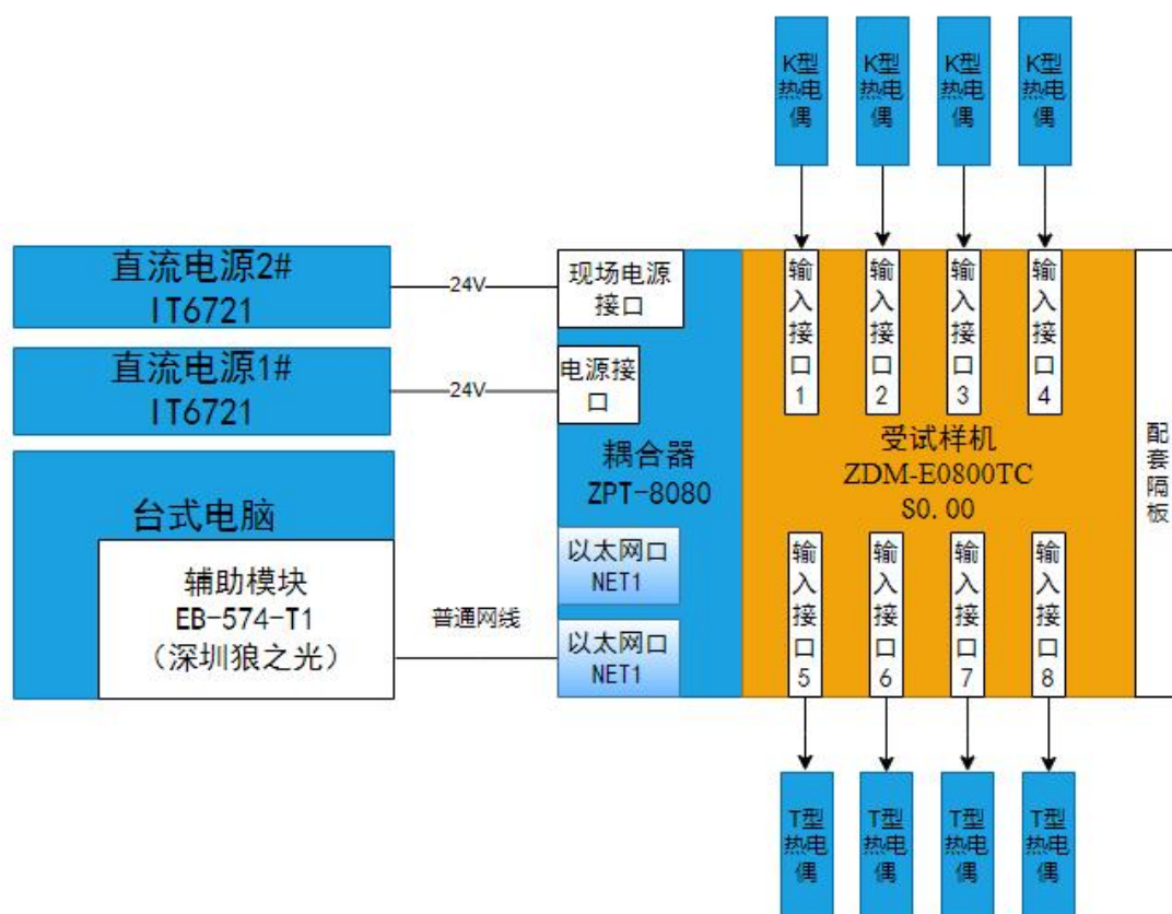
图 1 试验配置示意图
