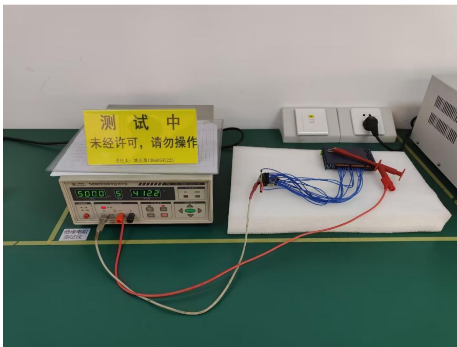
图2 绝缘电阻试验
