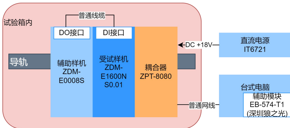
图 2 试验配置框图
