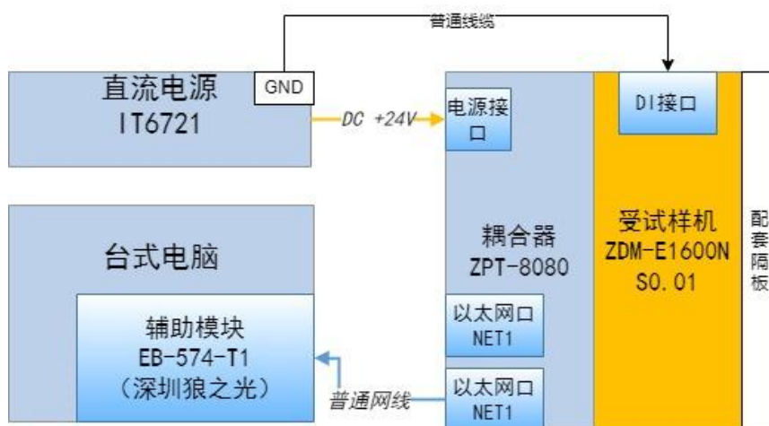
图 1 试验配置示意图
