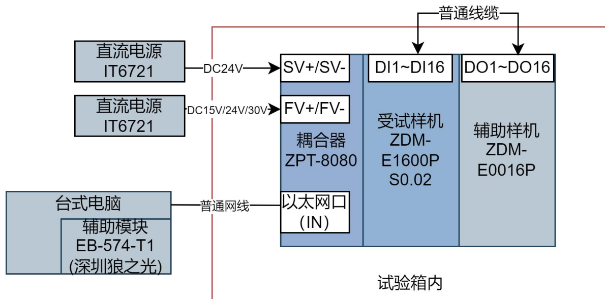
图 2 试验配置框图
