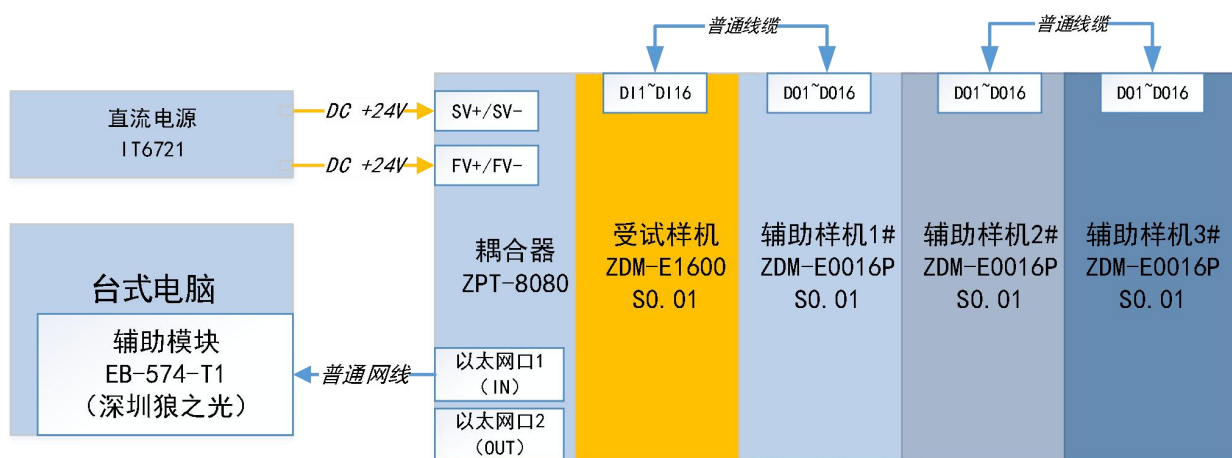
图 1 试验配置示意图
