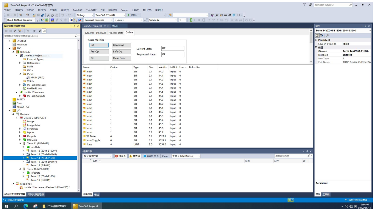
图 15 样机在湿热试验时第三次检查功能测试正常 (36VDC 供电)
