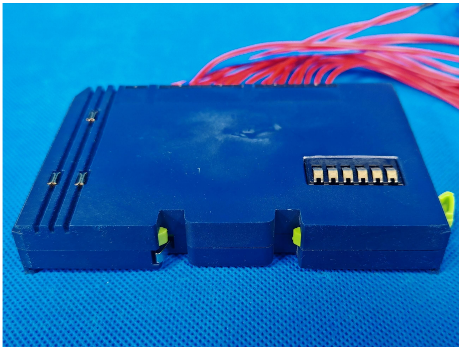
图 9 ZDM-E1600 后视图
