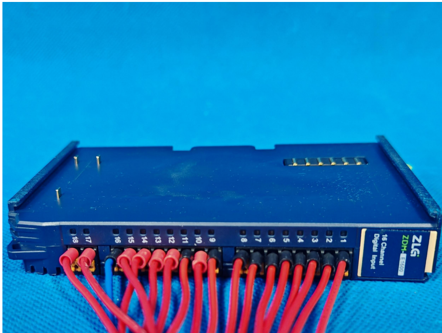
图 6 ZDM-E1600 正视图
