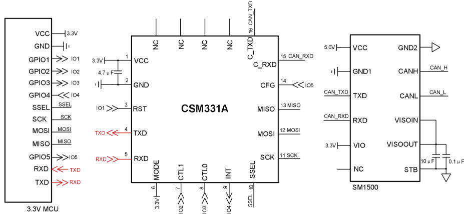
图 2.5 SPI 转 CAN 带错误反馈机制参考电路
