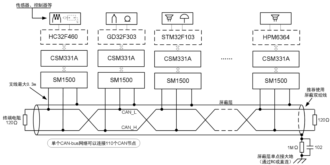
图 2.9 推荐组网示意图
