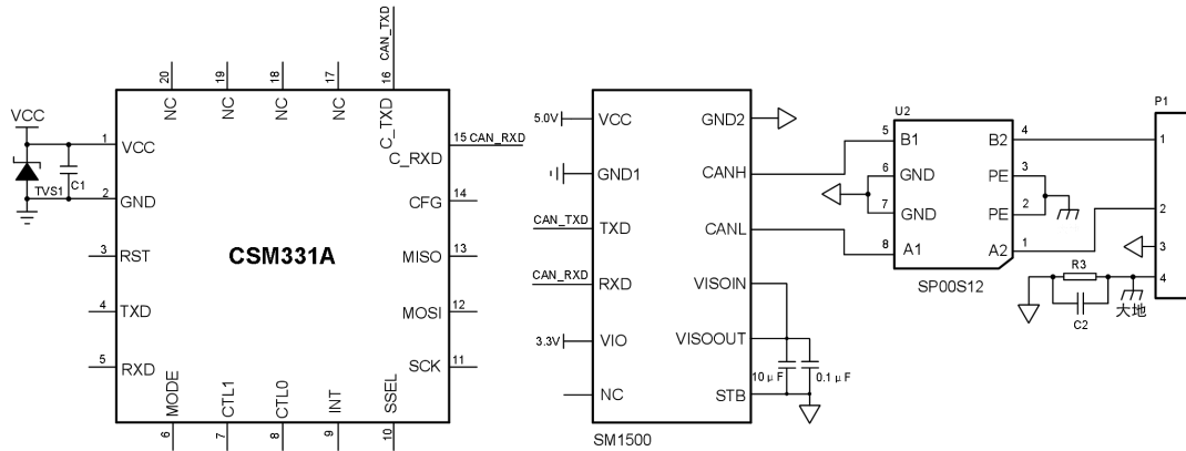
图 2.7 外围保护电路 1
