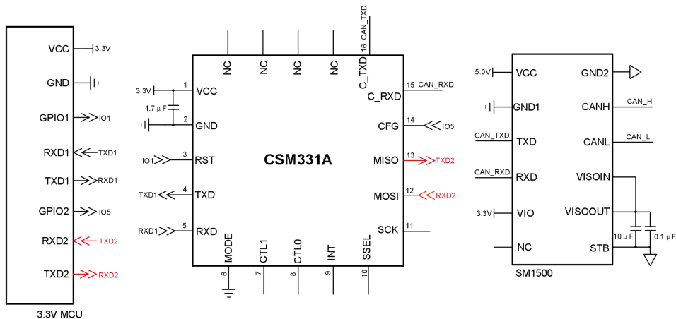
图 2.6 UART 转 CAN 带错误反馈机制参考电路
