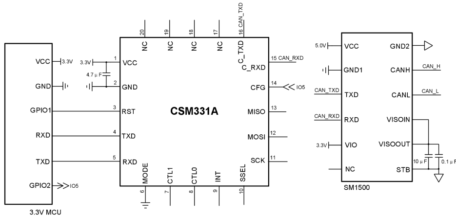
图 2.4 UART 转 CAN 参考电路
