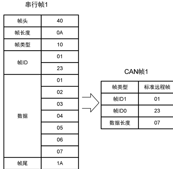
图 3.42 串行帧转 CAN 远程帧示例（自定义协议转换）
