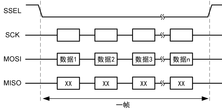
图 3.4 主机写数据帧示意
