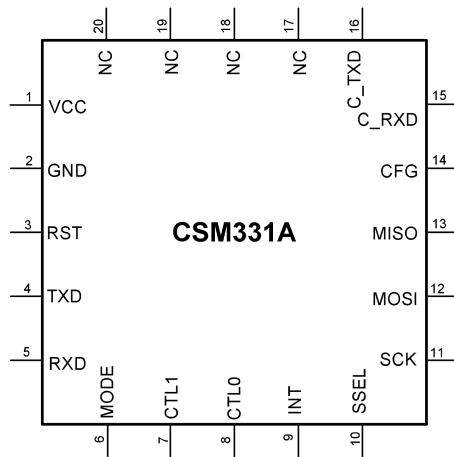
图 2.2 CSM331A 引脚排列
