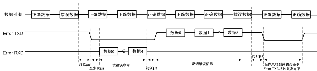
图 3.44 错误反馈机制时序图
