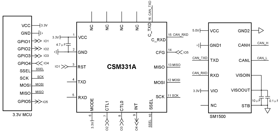
图 2.3 SPI 转 CAN 参考电路
