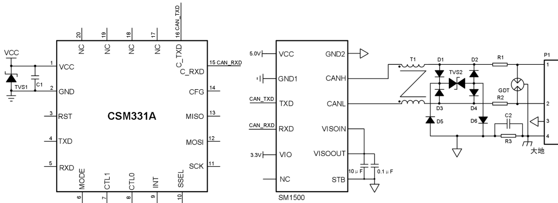
图 2.8 外围保护电路 2
