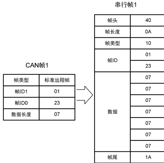
图 3.43 CAN 远程帧转串行帧示例（自定义协议转换）
