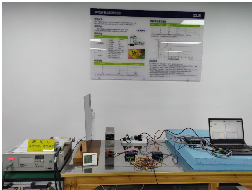
图 9 ESD 试验配置
