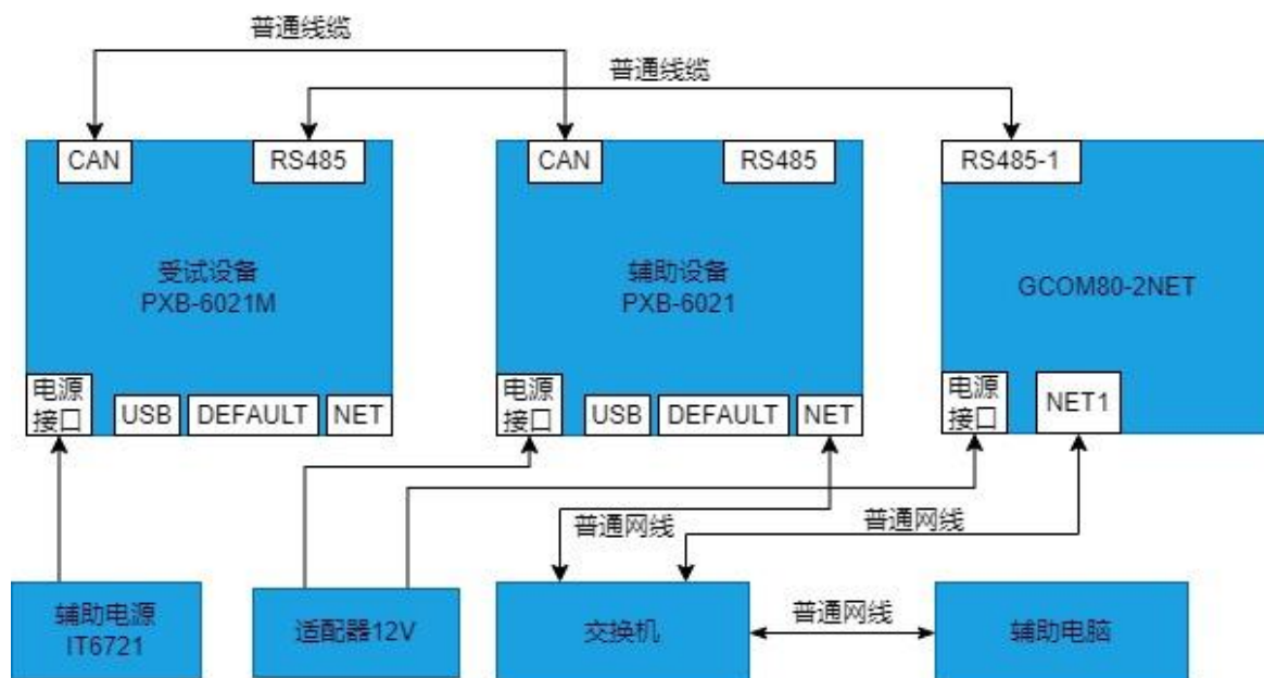
图 1 试验配置示意图
