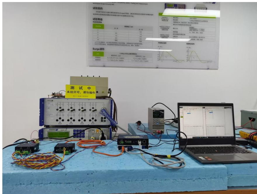
图 11 SURGE 试验配置
