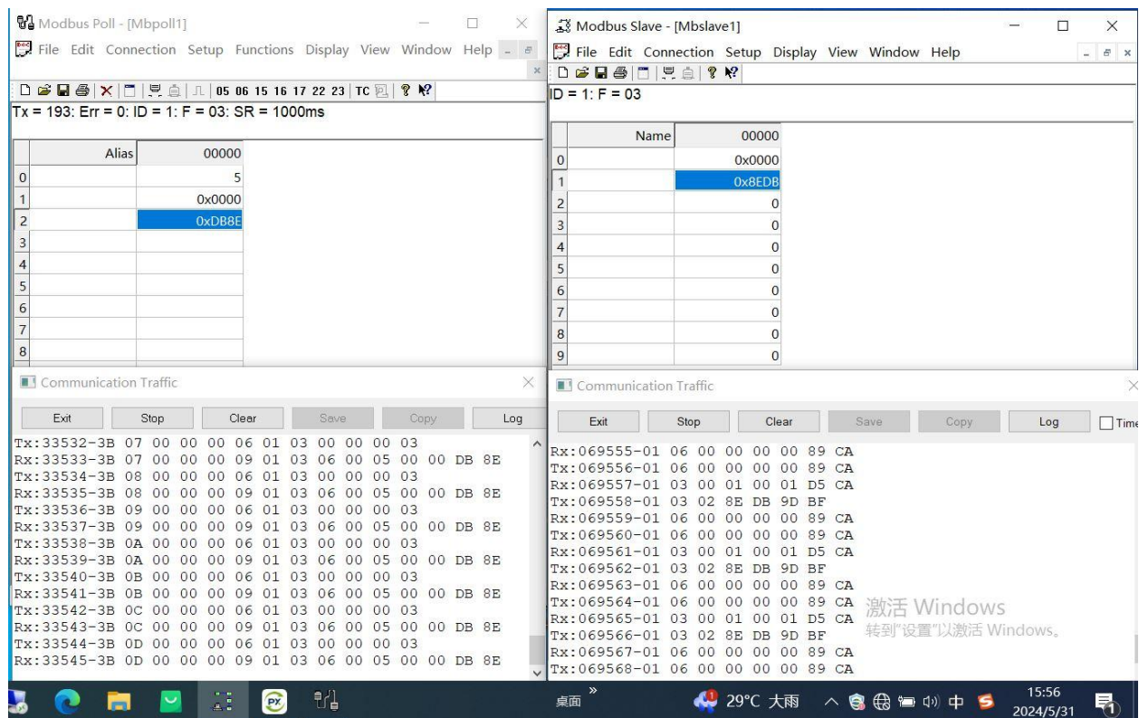
图 17 样机使用 RTU 协议时在+87°C第三次启动时功能测试正常
