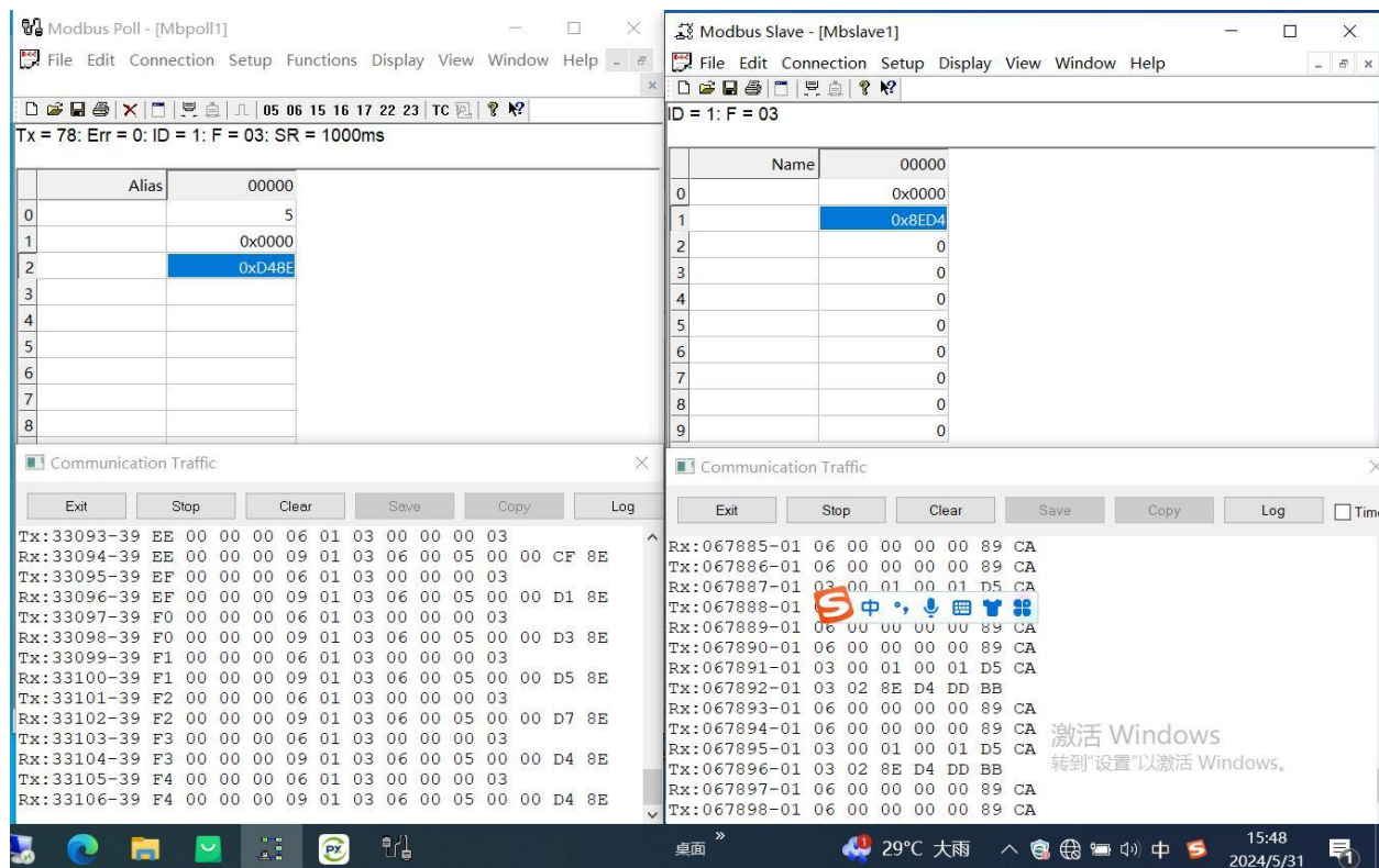
图 16 样机使用 RTU 协议时在+87°C第二次运行时功能测试正常
