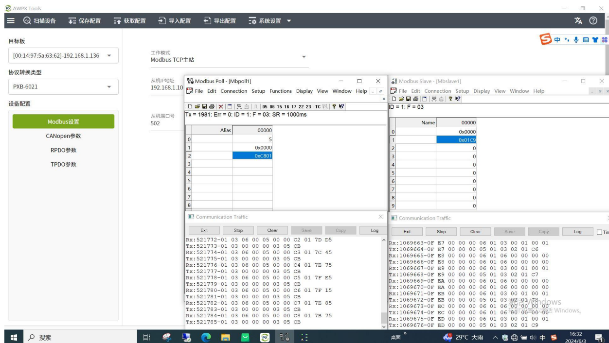
图 6 样机使用 TCP 协议时在-42℃第一次启动时功能测试正常
