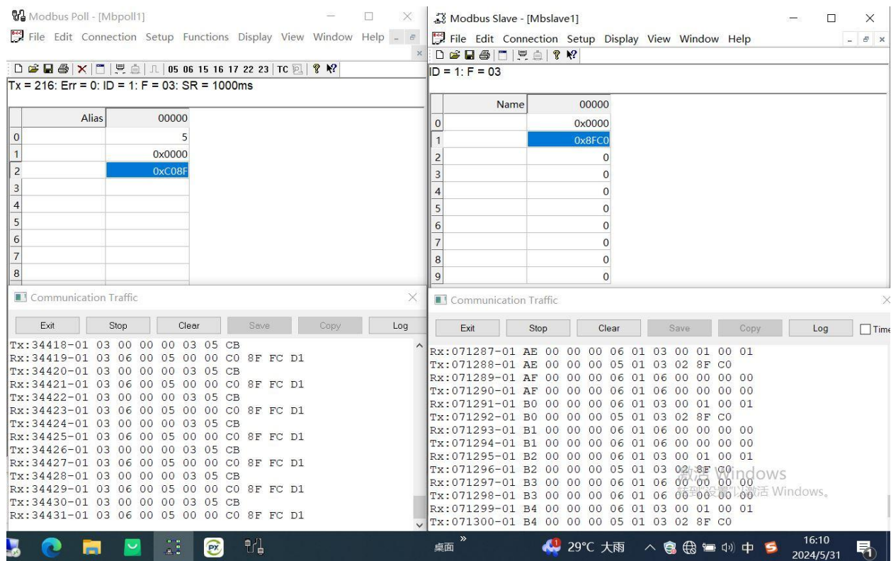
图 10 样机使用 TCP 协议时在+87℃第二运行时功能测试正常
