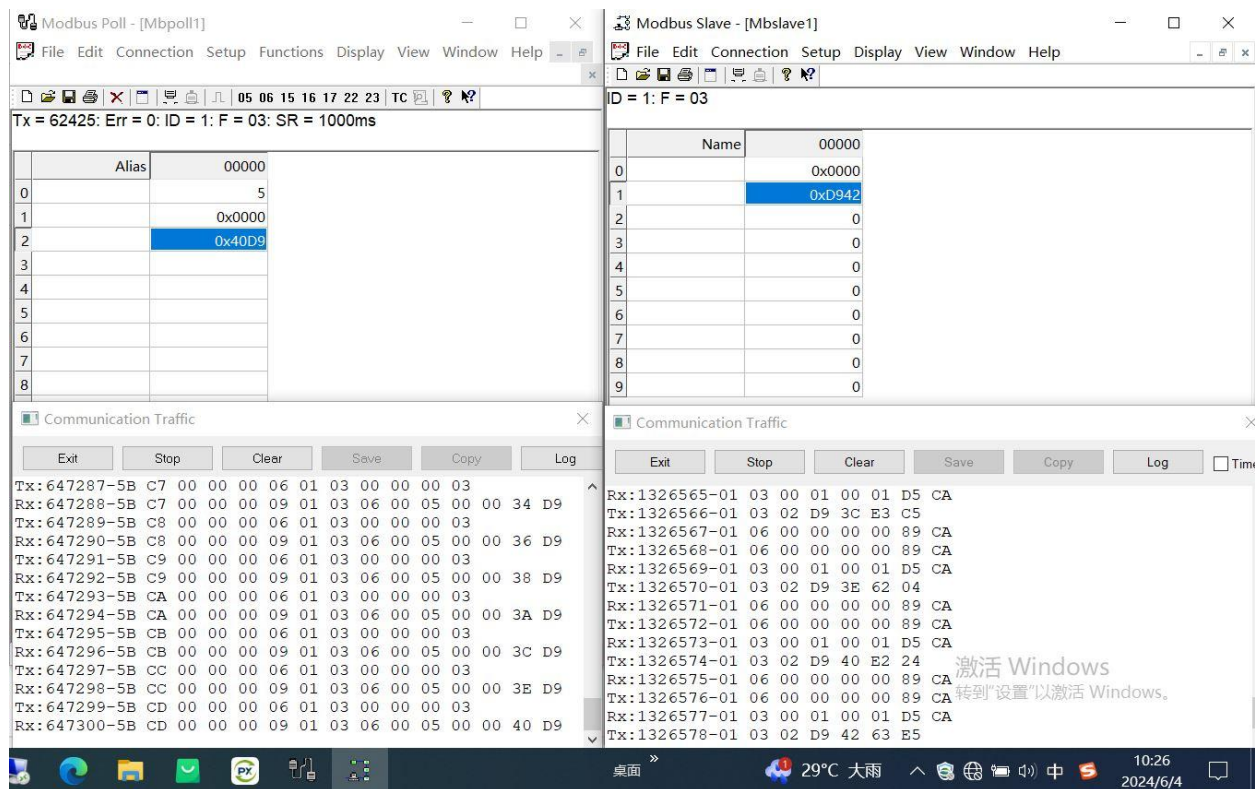
图 18 样机使用 RTU 协议时在温度变化时功能测试正常
