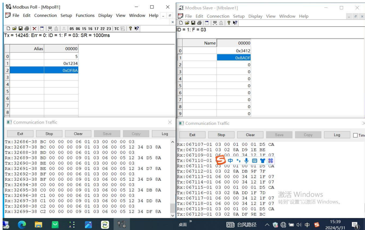
图 15 样机使用 RTU 协议时在+87°C第一次启动时功能测试正常
