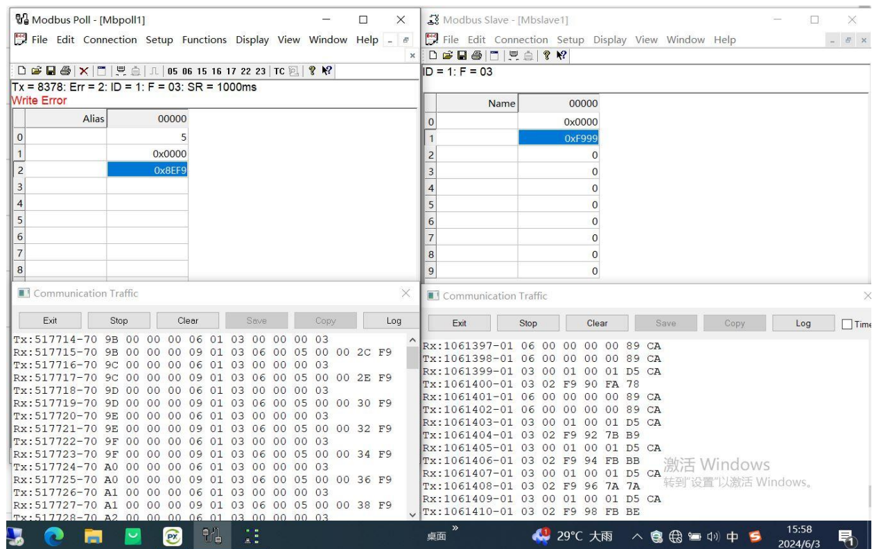
图 14 样机使用 RTU 协议时在-42°C第三次启动时功能测试正常
