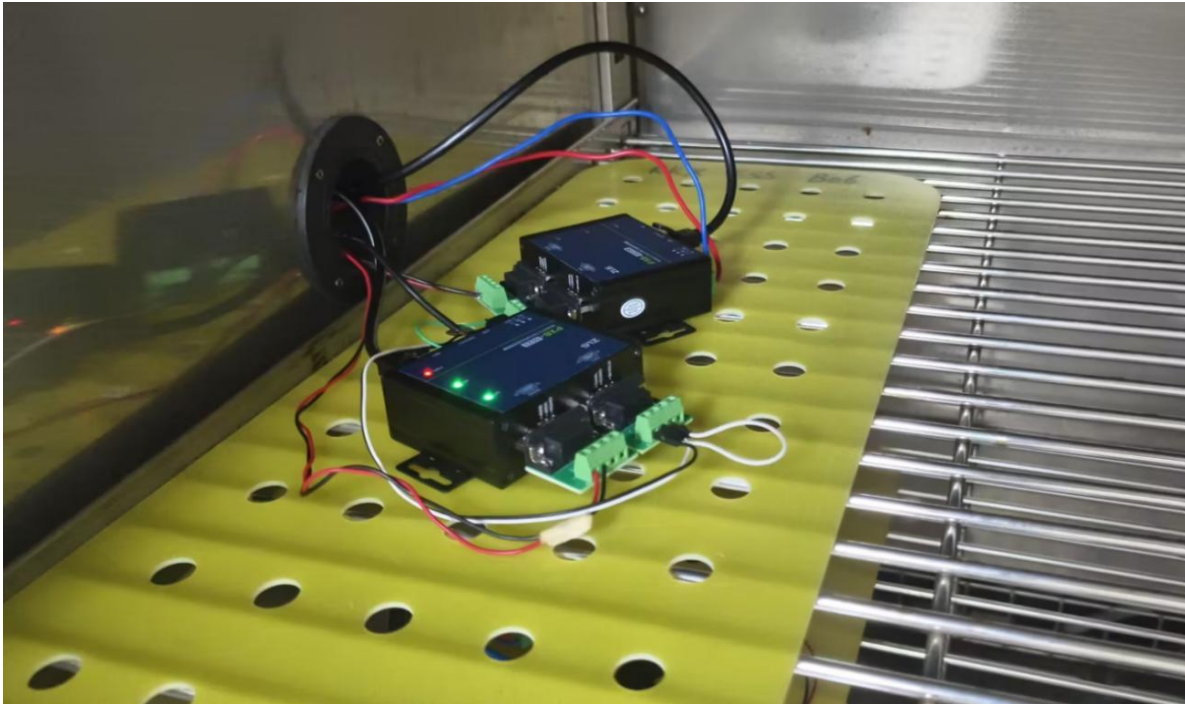
图 3 样机环境试验
