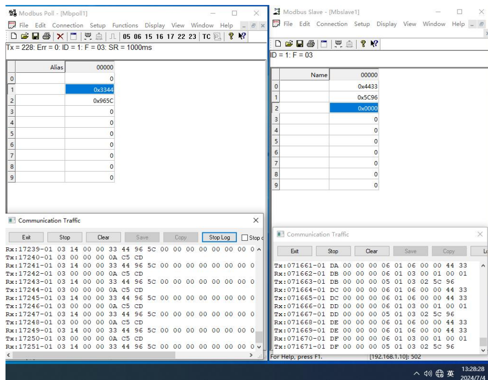
图 8 样机在高温试验时第二次启动运行检查功能正常 (RTU 模式, 供电电压 9VDC)
