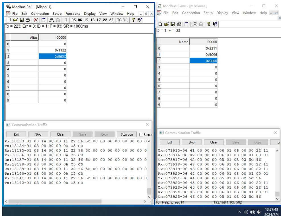
图 9 样机在高温试验时第三次启动运行检查功能正常（RTU 模式，供电电压 36VDC）
