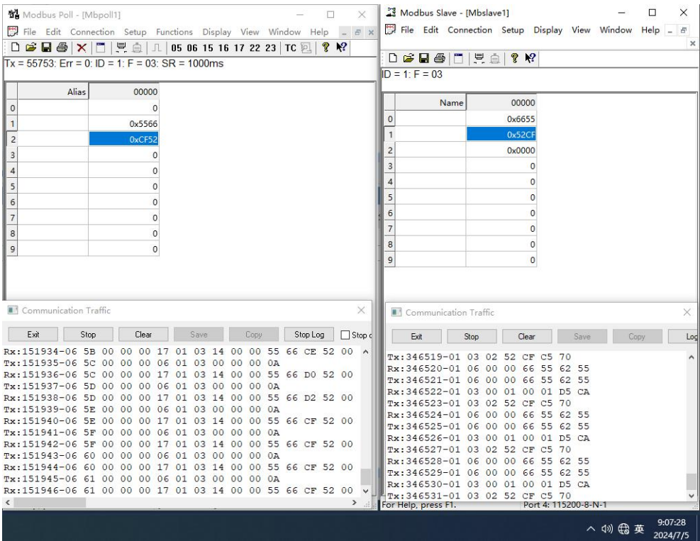
图 13 样机在湿热试验时过程运行检查功能正常（TCP 模式，供电电压 12VDC）
