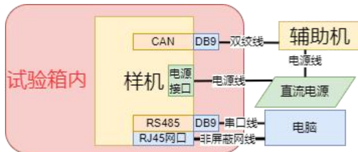
图 2 试验配置框图
