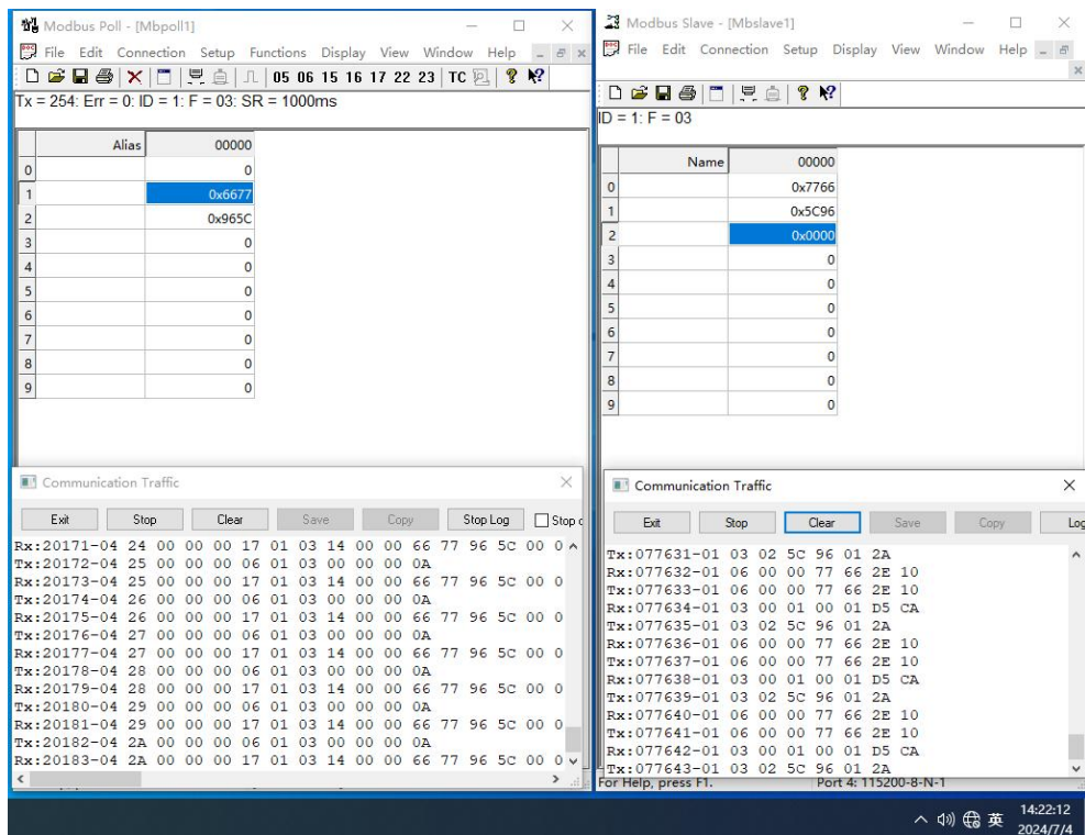
图 11 样机在高温试验时第五次启动运行检查功能正常（TCP 模式，供电电压 12VDC）
