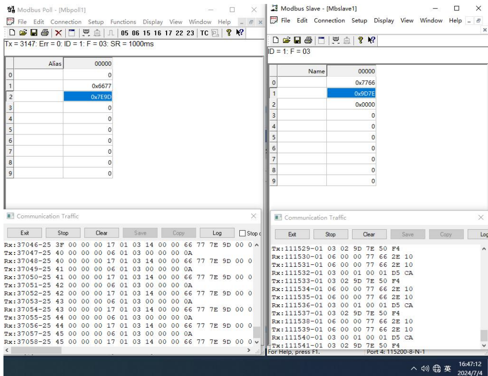
图 12 样机在高温试验时第六次启动运行检查功能正常（TCP 模式，供电电压 9VDC）
