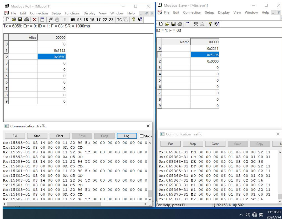
图 7 样机在高温试验时第一次启动运行检查功能正常 (RTU 模式, 供电电压 12VDC)
