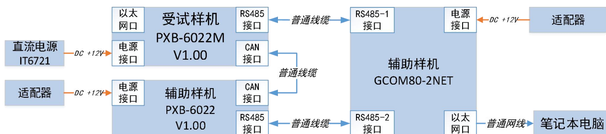
图 1 试验配置①网络连接示意图
