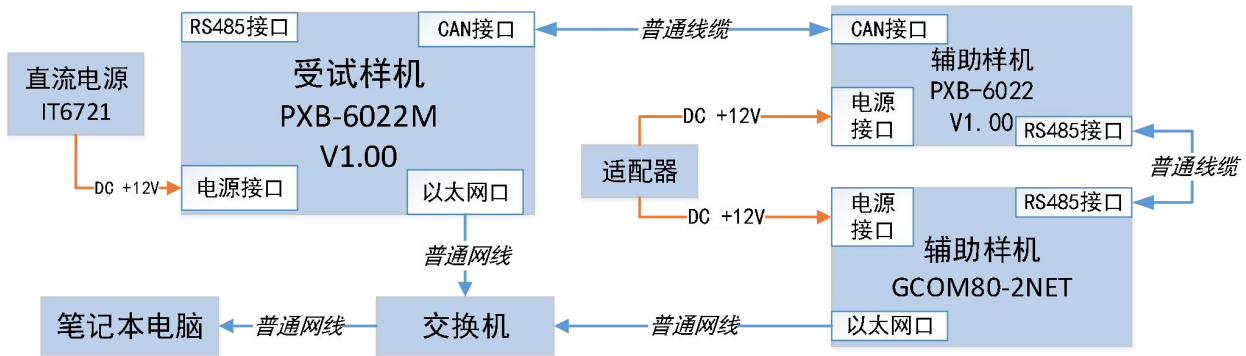
图 3 试验配置②网络连接示意图
