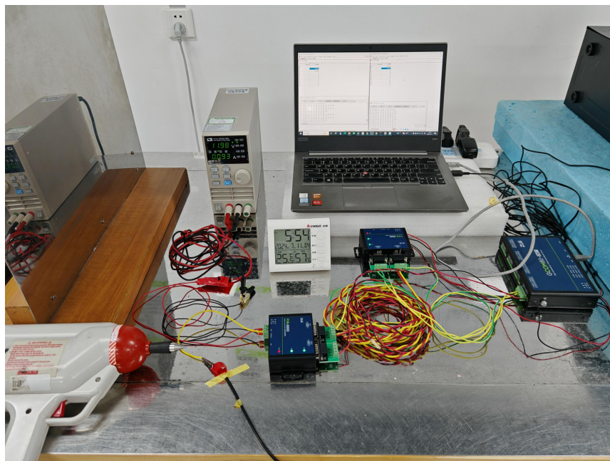
图 10 试验配置①ESD 试验现场配置图
