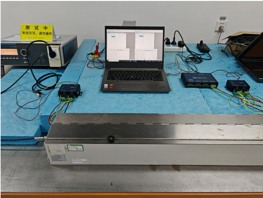
图 12 试验配置①的 EFT 试验现场配置图
