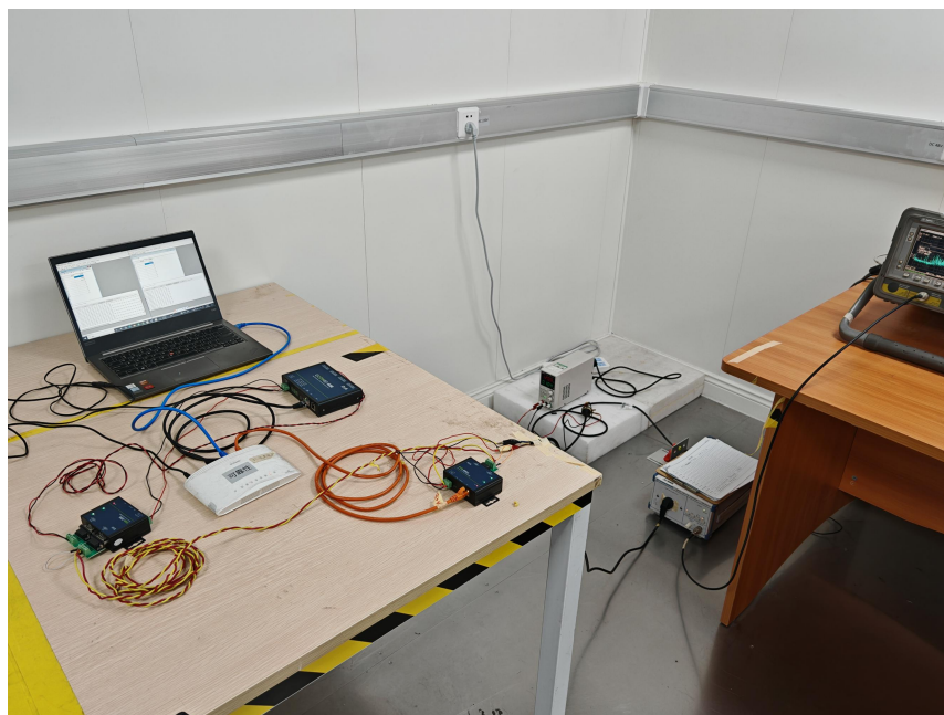
图 15 试验配置②的 CE 试验现场配置图
