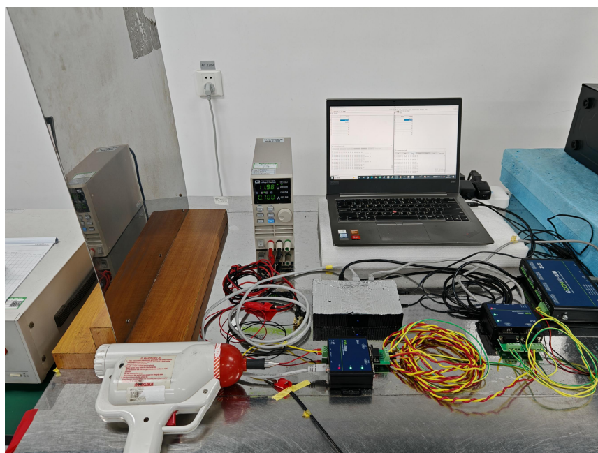
图 11 试验配置②ESD 试验现场配置图
