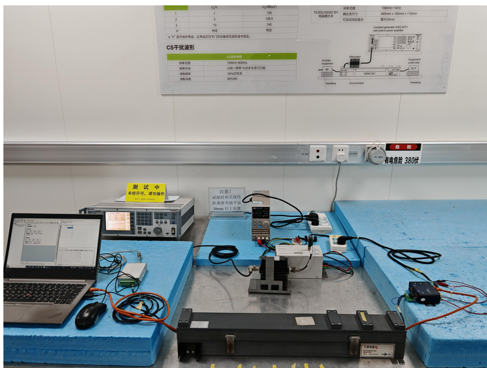
图 11 试验配置②CS 试验现场图
