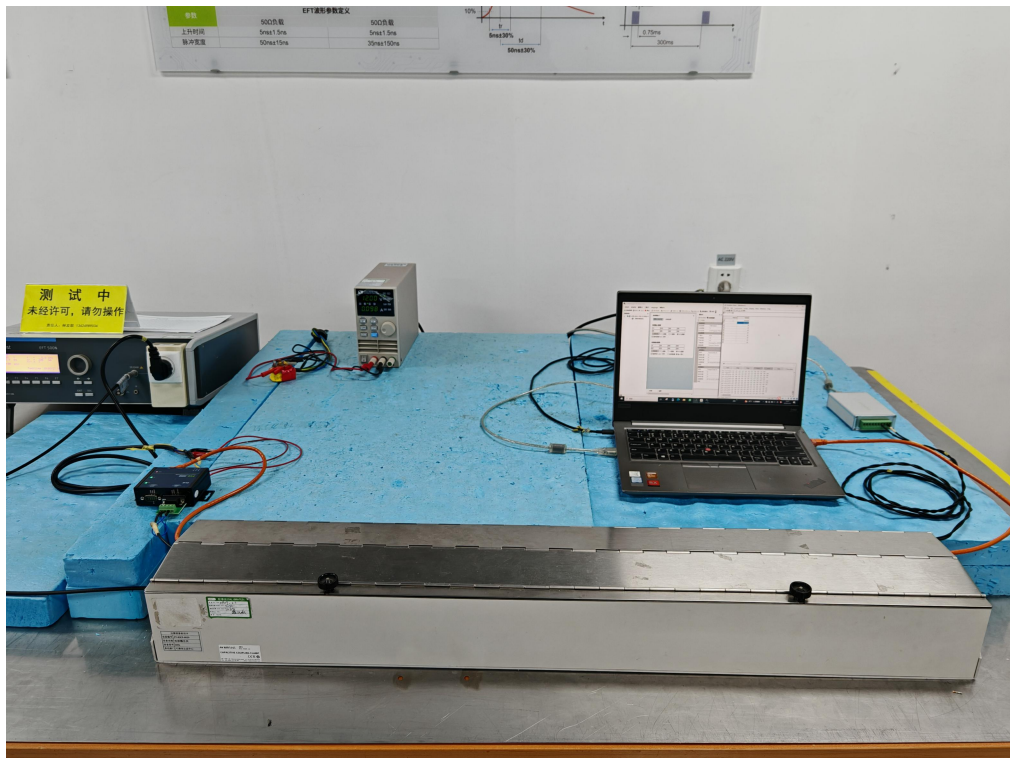
图 7 EFT 试验配置②现场配置图
