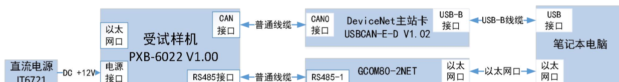
图 1 试验配置①示意图
