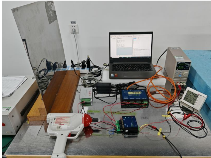
图 3 ESD 试验配置①现场图
