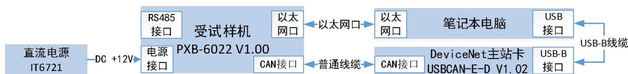
图 2 试验配置②示意图
