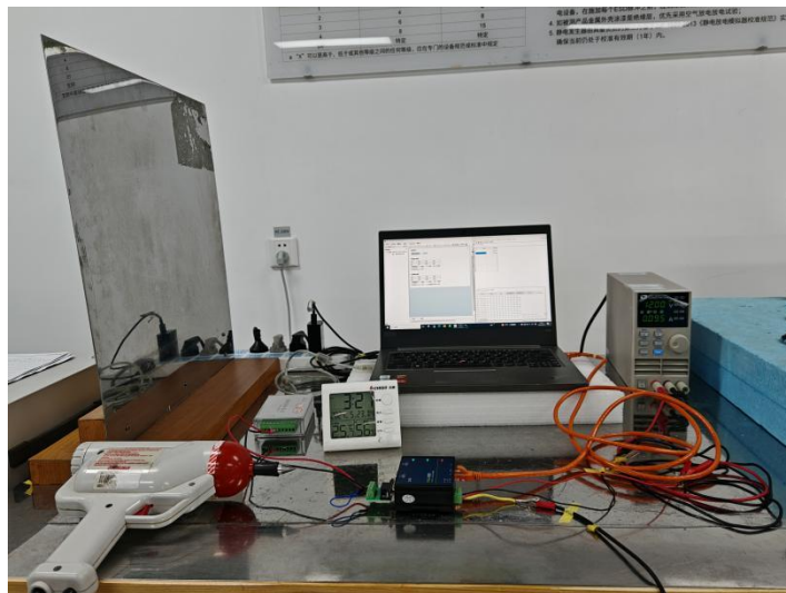
图 4 ESD 试验配置②现场图
