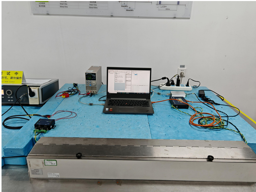
图 6 EFT 试验配置①现场配置图
