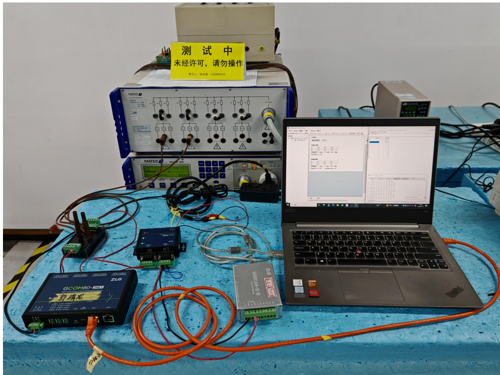
图 8 试验配置①浪涌试验现场图
