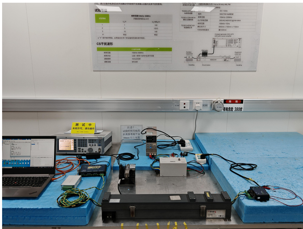
图 10 试验配置①CS 试验现场图
