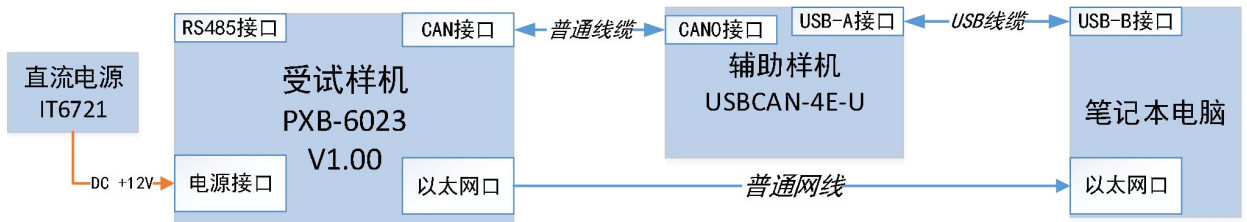
图 3 试验配置②网络连接示意图
