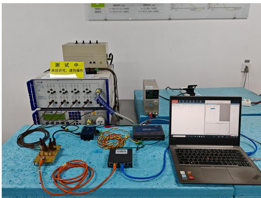
图 15 试验配置②的浪涌试验现场配置图
