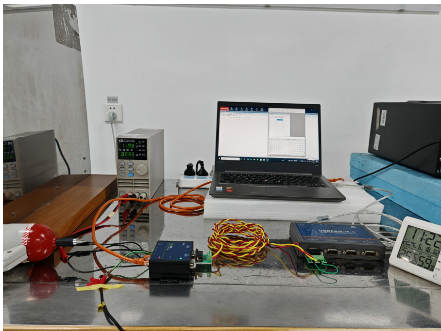
图 11 试验配置②ESD 试验现场配置图
