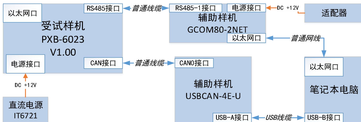
图 1 试验配置①网络连接示意图
