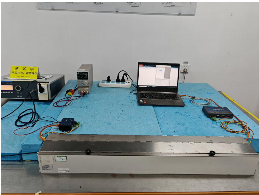
图 13 试验配置②的 EFT 试验现场配置图
