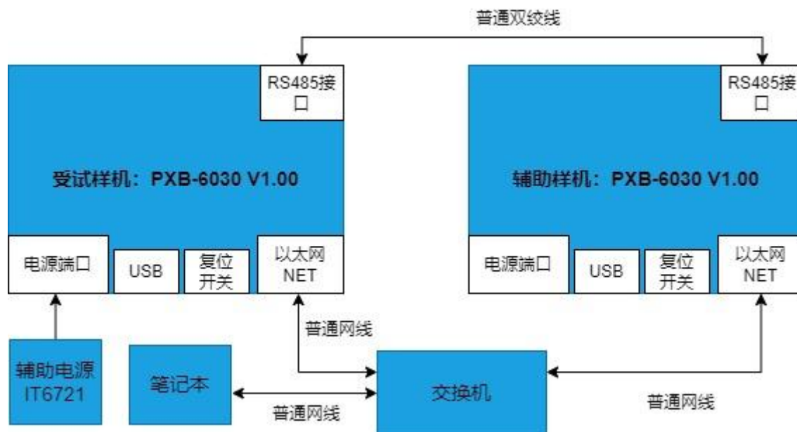
图 1 试验配置示意图
