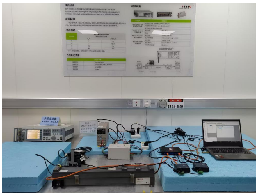
图 8 CS 试验配置
