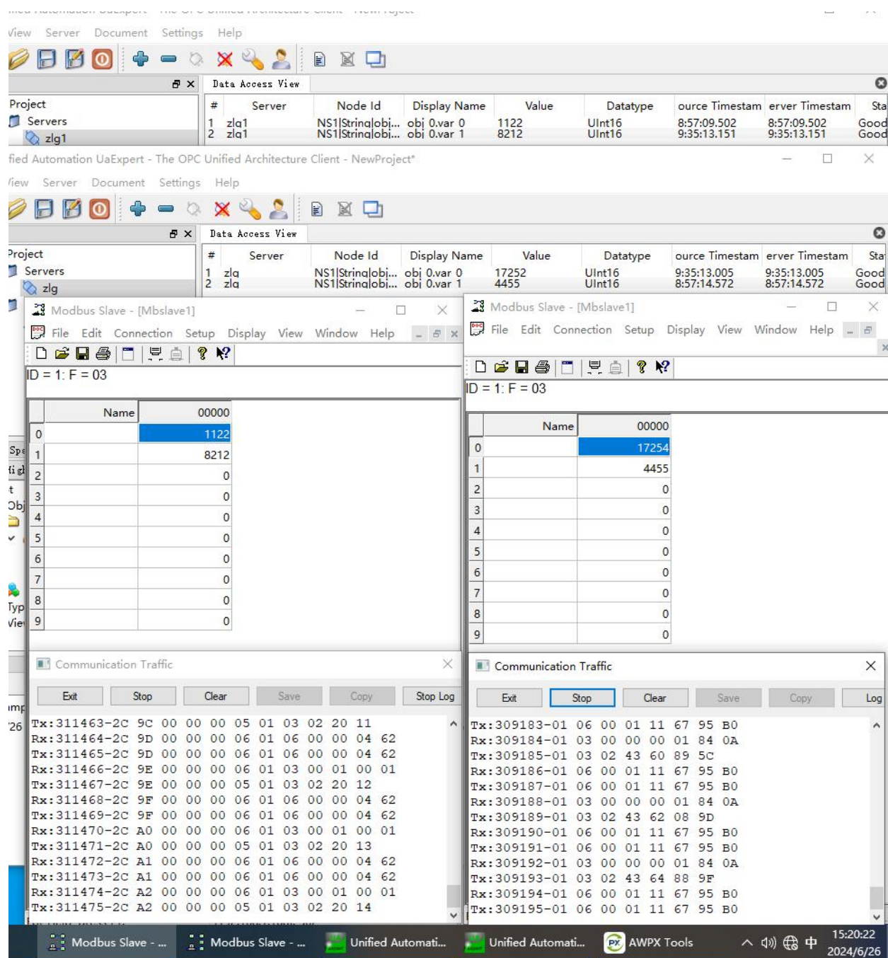
图 9 样机在低温试验时第三次启动运行检查功能正常（供电电压 9VDC）
