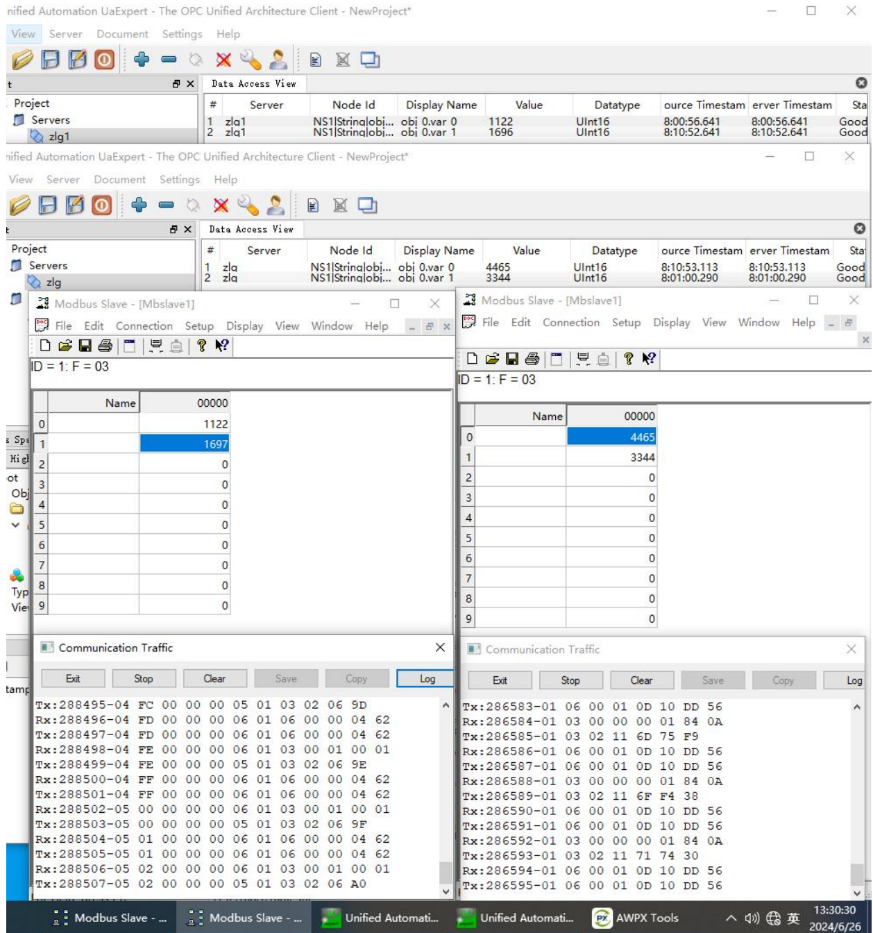
图 8 样机在低温试验时第二次启动运行检查功能正常（供电电压 12VDC）
