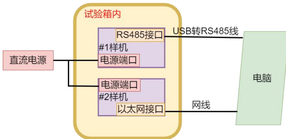
图 2 试验配置框图
