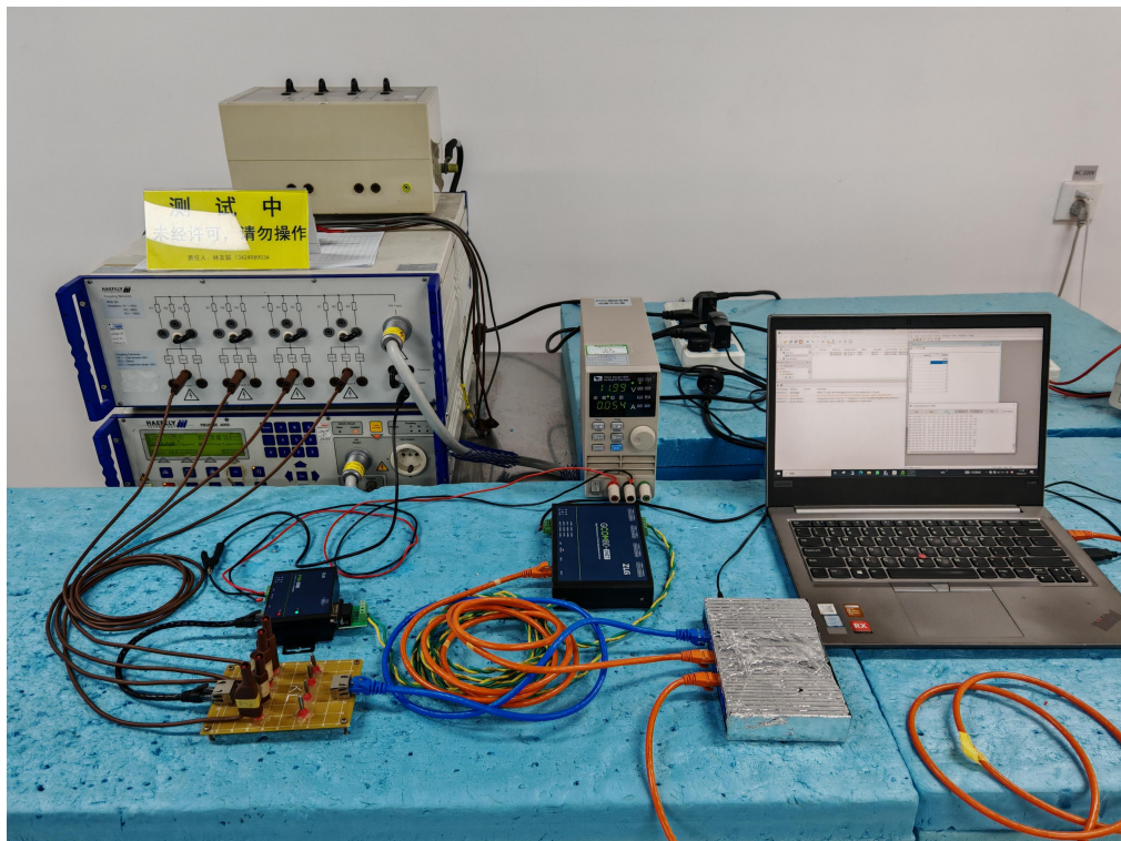
图 4 浪涌试验现场配置图（信号接口）
