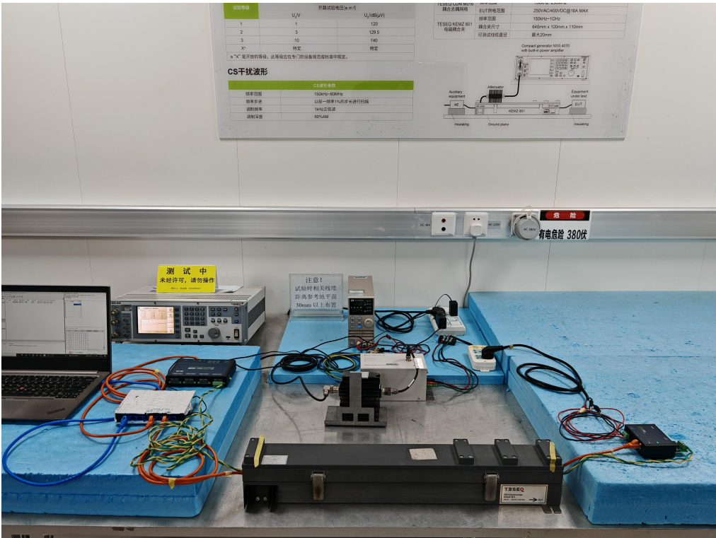
图 5 CS 试验现场配置图
