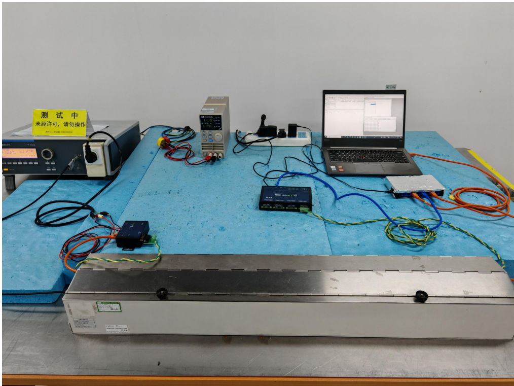
图 2 EFT 试验现场配置图
