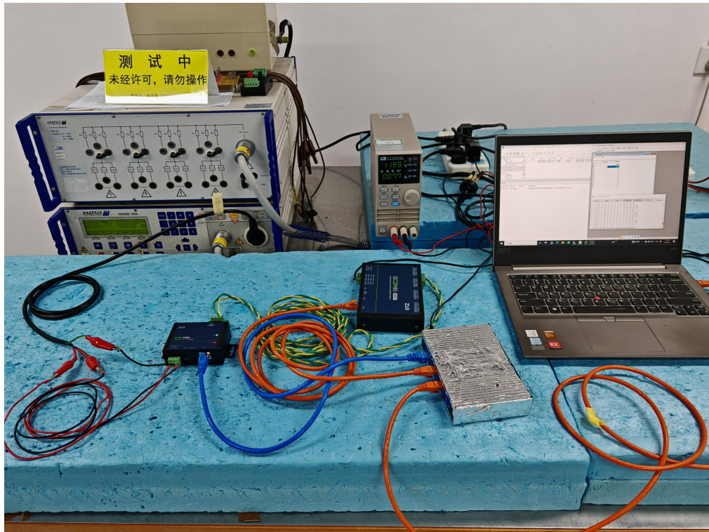
图 3 浪涌试验现场配置图（电源接口）
