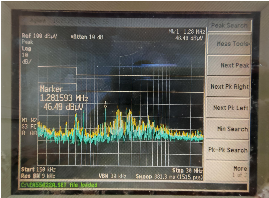
EUT-N 线 (QP&AVG 值)
