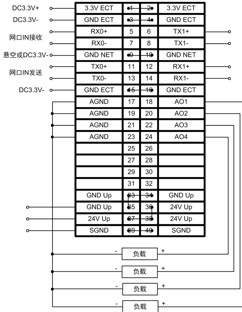
图 4.3 ZIOC-E0004A/ZIOC-E0004A11 典型接线图
