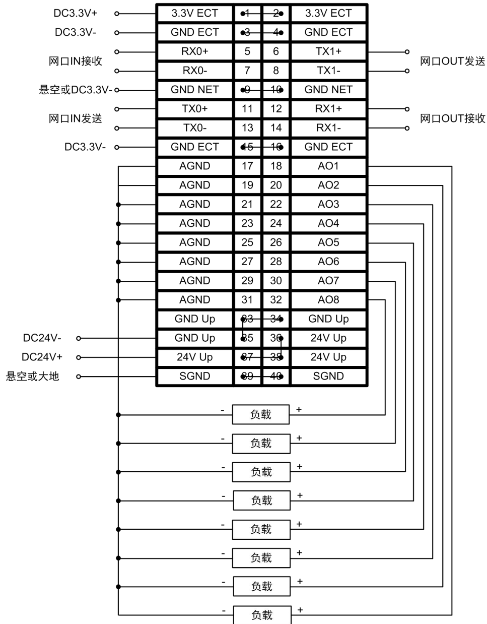
图 4.1 ZIOC-E0008AU 典型接线图
