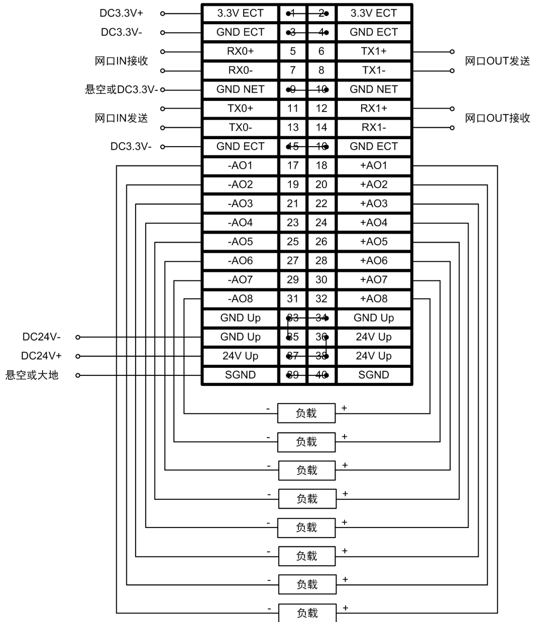
图 4.2 ZIOC-E0008AU1 典型接线图
