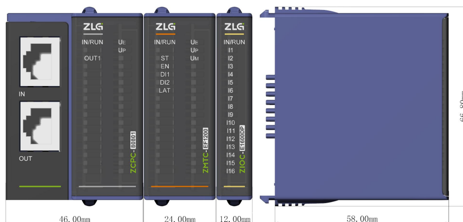
图 3.1 尺寸图
