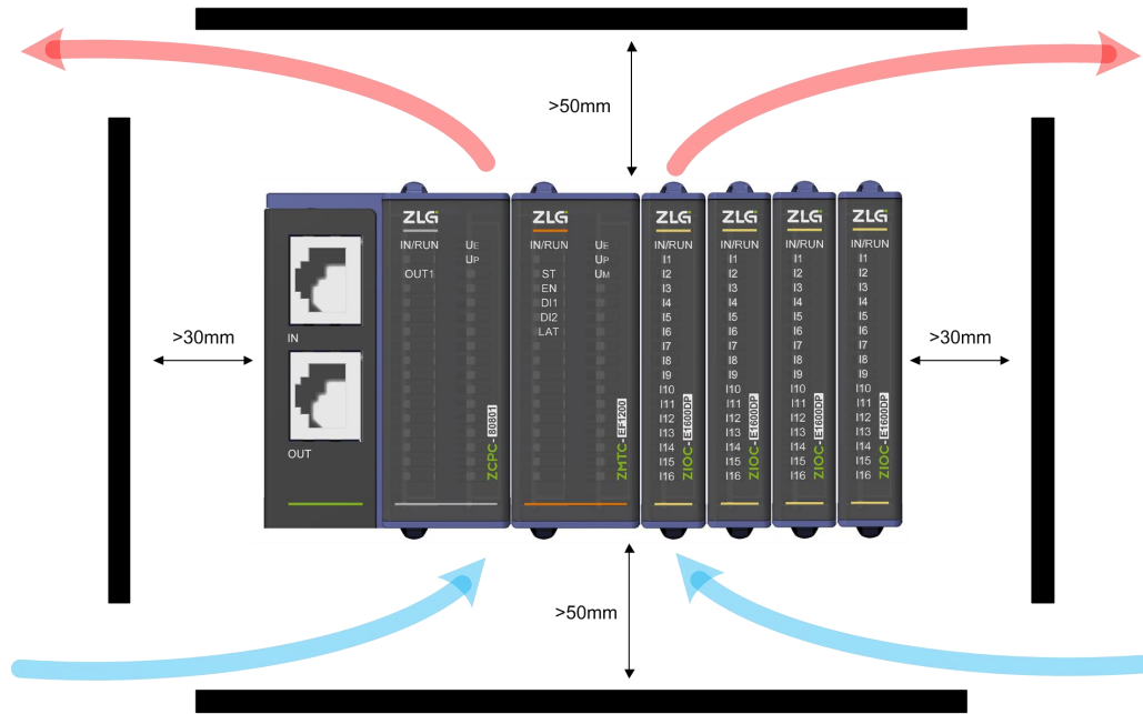
图 3.4 散热空间
