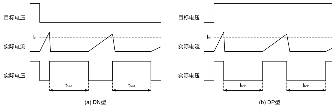
图 6.1 过流保护
