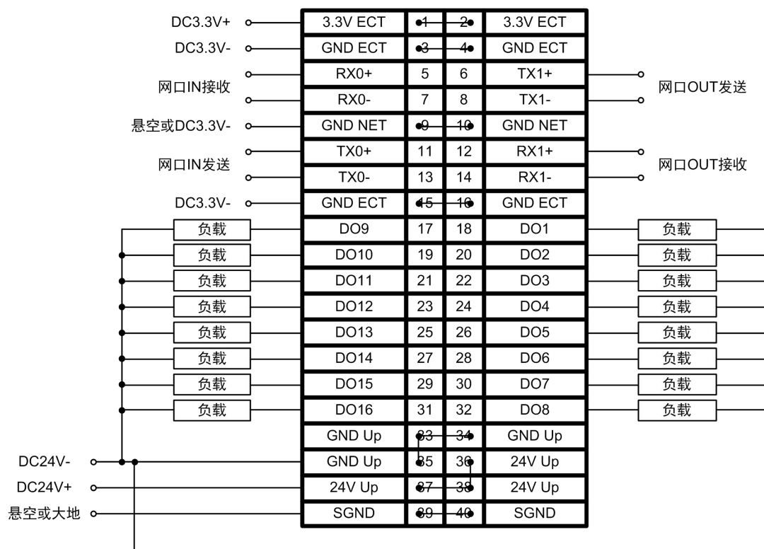
图 4.2 ZIOC-E0016DP 典型接线图
