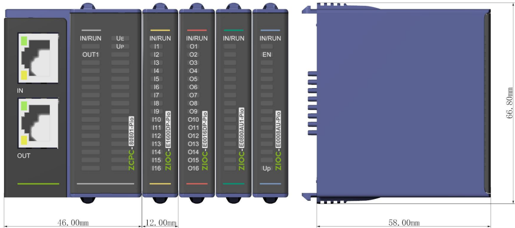
图 3.1 尺寸图
