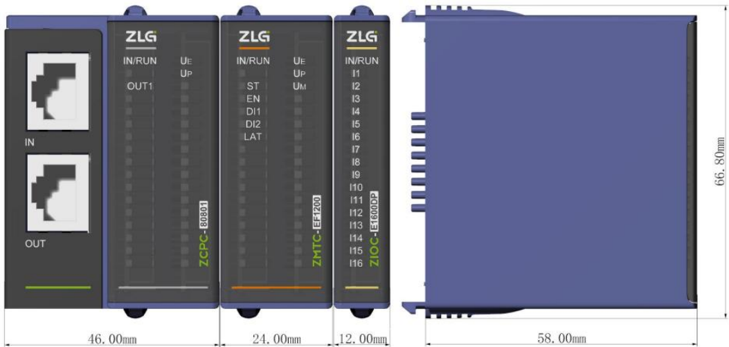
图 3.1 尺寸图
