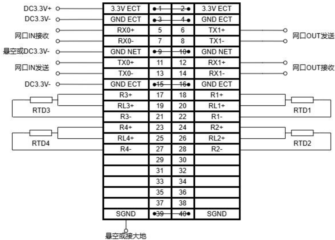
图 4.1 ZIOC-E0400P3 典型接线图
